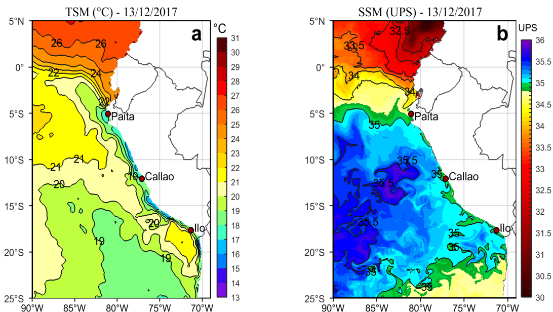
Figura 2. a) Temperatura superficial del mar ( ^{\circ}\text{C} ) y b) Salinidad superficial del mar (UPS) para el 13 de diciembre. Datos: OSTIA-UKMO-L4-GLOB-v2.0 (UK Met Office, 2012; Donlon et al, 2012) disponible en https://podaac.jpl.nasa.gov/dataset/OSTIA-UKMO-L4-GLOB-v2.0 para (a) y Hybrid Coordinate Ocean Model (HYCOM; Halliwell et al., 1998; 2000; Bleck, 2001) para (b). Procesamiento: LHF/AFIOF/DGIOCC/IMARPE.
