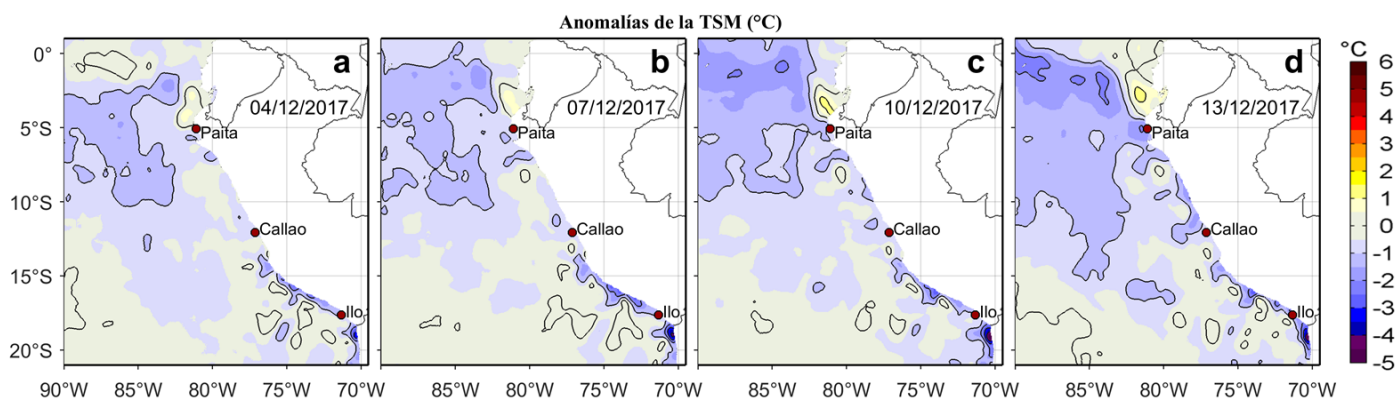
Figura 3. Anomalías de la Temperatura Superficial del Mar ( ^{\circ}\text{C} ) para los días: a) 04, b) 07, c) 10 y d) 13 de diciembre de 2017. Las anomalías se calcularon respecto de la climatología para el periodo 2007-2016. Datos: OSTIA-UKMO-L4-GLOB-v2.0 (UK Met Office, 2012; Donlon et al, 2012). Procesamiento: LHF/AFIOF/DGIOCC/IMARPE.
