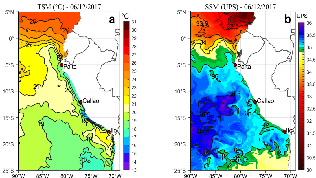
Figura 2. a) Temperatura superficial del mar ( ^{\circ}\text{C} ) y b) Salinidad superficial del mar (UPS) para el 06 de diciembre. Datos: OSTIA-UKMO-L4-GLOB-v2.0 (UK Met Office, 2012; Donlon et al, 2012) disponible en https://podaac.jpl.nasa.gov/dataset/OSTIA-UKMO-L4-GLOB-v2.0 para (a) y Hybrid Coordinate Ocean Model (HYCOM; Halliwell et al., 1998; 2000; Bleck, 2001) para (b). Procesamiento: LHF/AFIOF/DGIOCC/IMARPE.
