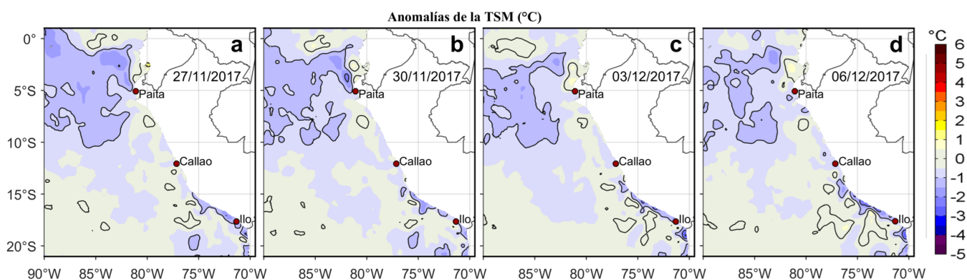
Figura 3. Anomalías de la Temperatura Superficial del Mar ( ^{\circ}\text{C} ) para los días: a) 27 y b) 30 de noviembre, c) 03, y d) 06 de diciembre de 2017. Las anomalías se calcularon respecto de la climatología para el periodo 2007-2016. Datos: OSTIA-UKMO-L4-GLOB-v2.0 (UK Met Office, 2012; Donlon et al, 2012). Procesamiento: LHF/AFIOF/DGIOCC/IMARPE.
