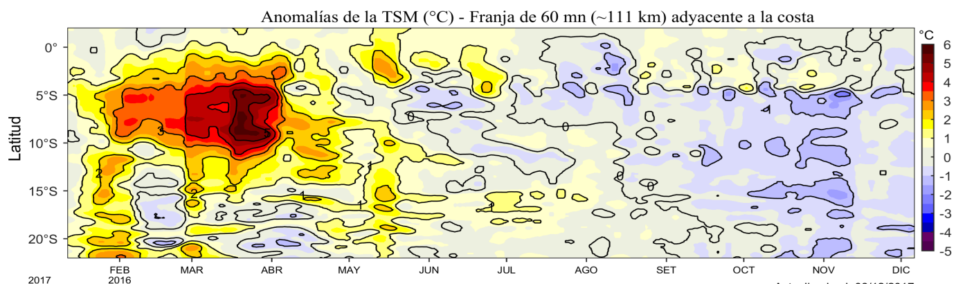
Figura 4. Variación promedio de las anomalías de la temperatura superficial del mar ( ^{\circ}\text{C} ) para una franja de 60 mn ( \sim 111 km) adyacente a la costa para los últimos doce meses al 06 de diciembre de 2017. Datos: OSTIA-UKMO-L4-GLOB-v2.0 (UK Met Office, 2012; Donlon et al, 2012) disponible en https://podaac.jpl.nasa.gov/dataset/OSTIA-UKMO-L4-GLOB-v2.0 . Las anomalías se calcularon con respecto al periodo 2007-2016. Procesamiento: LHF/AFIOF/DGIOCC/IMARPE.
