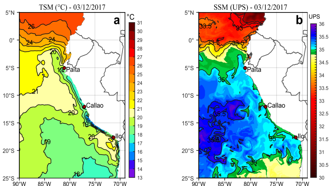
Figura 2. a) Temperatura superficial del mar ( ^{\circ}\text{C} ) y b) Salinidad superficial del mar (UPS) para el 03 de diciembre. Datos: OSTIA-UKMO-L4-GLOB-v2.0 (UK Met Office, 2012; Donlon et al, 2012) disponible en https://podaac.jpl.nasa.gov/dataset/OSTIA-UKMO-L4-GLOB-v2.0 para (a) y Hybrid Coordinate Ocean Model (HYCOM; Halliwell et al., 1998; 2000; Bleck, 2001) para (b). Procesamiento: LHF/AFIOF/DGIOCC/IMARPE.
