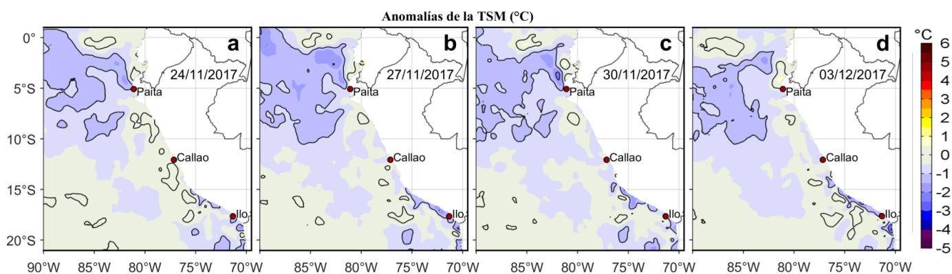
Figura 3. Anomalías de la Temperatura Superficial del Mar ( ^{\circ}\text{C} ) para los días: a) 24, b) 27 y c) 30 de noviembre y d) 03 de diciembre de 2017. Las anomalías se calcularon respecto de la climatología para el periodo 2007-2016. Datos: OSTIA-UKMO-L4-GLOB-v2.0 (UK Met Office, 2012; Donlon et al, 2012). Procesamiento: LHF/AFIOF/DGIOCC/IMARPE.
