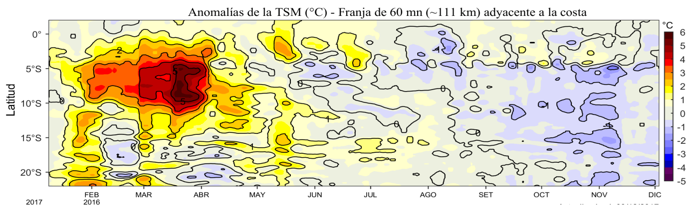
Figura 4. Variación promedio de las anomalías de la temperatura superficial del mar ( ^{\circ}\text{C} ) para una franja de 60 mn ( \sim 111 km) adyacente a la costa para los últimos doce meses al 03 de diciembre de 2017. Datos: OSTIA-UKMO-L4-GLOB-v2.0 (UK Met. Office, 2012; Donlon et al, 2012) disponible en https://podaac.jpl.nasa.gov/dataset/OSTIA-UKMO-L4-GLOB-v2.0 . Las anomalías se calcularon con respecto al periodo 2007-2016. Procesamiento: LHF/AFIOF/DGIOCC/IMARPE.
