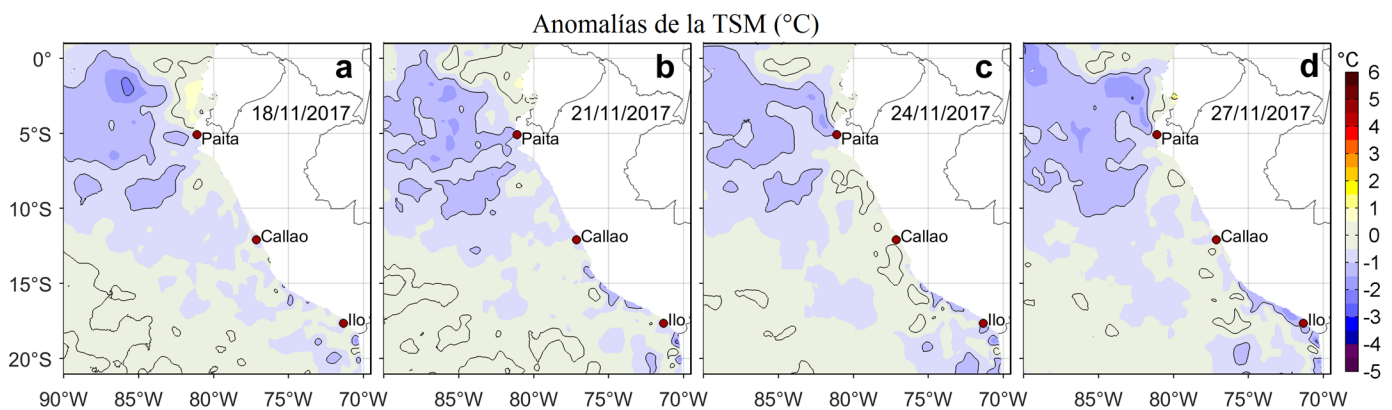
Figura 3. Anomalías de la Temperatura Superficial del Mar ( ^{\circ}\text{C} ) para los días: a) 18, b) 21, c) 24, y d) 27 de noviembre de 2017. Las anomalías se calcularon respecto de la climatología para el periodo 2007-2016. Datos: OSTIA-UKMO-L4-GLOB-v2.0 (UK Met Office, 2012; Donlon et al, 2012). Procesamiento: LHF/AFIOF/DGIOCC/IMARPE.
