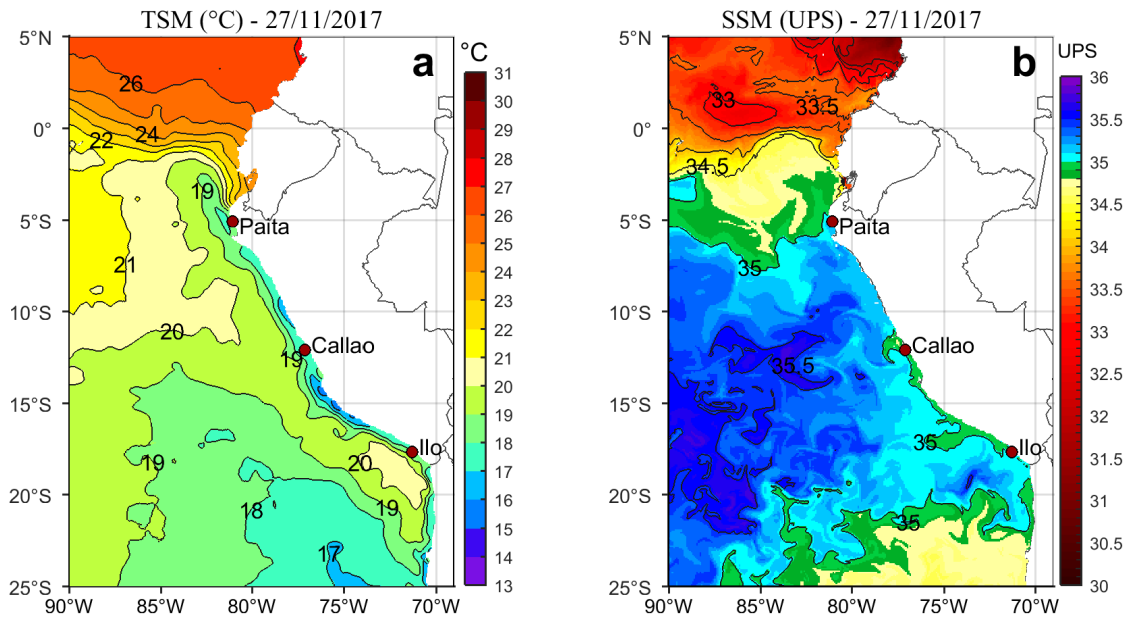
Figura 2. a) Temperatura superficial del mar ( ^{\circ}\text{C} ) y b) Salinidad superficial del mar (UPS) para el 27 de noviembre. Datos: OSTIA-UKMO-L4-GLOB-v2.0 (UK Met Office, 2012; Donlon et al, 2012) disponible en https://podaac.jpl.nasa.gov/dataset/OSTIA-UKMO-L4-GLOB-v2.0 para (a) y Hybrid Coordinate Ocean Model (HYCOM; Halliwell et al., 1998; 2000; Bleck, 2001) para (b). Procesamiento: LHF/AFIOF/DGIOCC/IMARPE.
