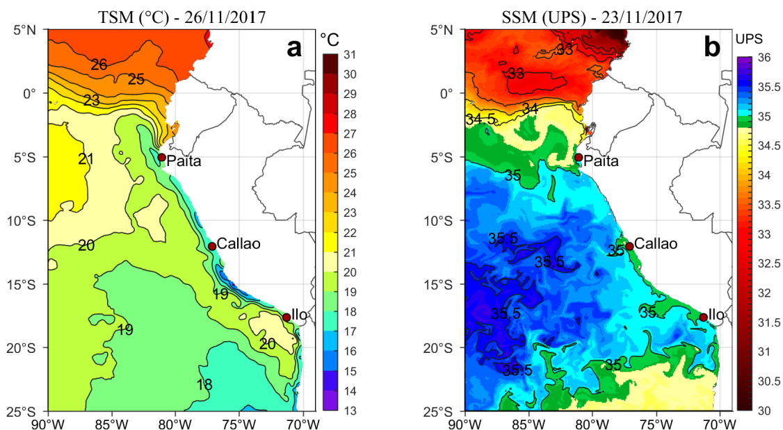
Figura 2. a) Temperatura superficial del mar (°C) y b) Salinidad superficial del mar (UPS) para el 26 de noviembre y 23 de noviembre, respectivamente. Datos: OSTIA-UKMO-L4-GLOB-v2.0 (UK Met Office, 2012; Donlon et al, 2012) disponible en https://podaac.jpl.nasa.gov/dataset/OSTIA-UKMO-L4-GLOB-v2.0 para (a) y Hybrid Coordinate Ocean Model (HYCOM; Halliwell et al.,
