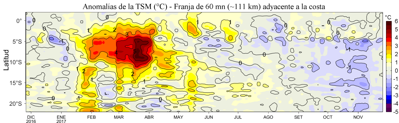
Figura 4. Variación promedio de las anomalías de la temperatura superficial del mar (°C) para una franja de 60 mn (~111 km) adyacente al litoral peruano para los últimos doce meses al 26 de noviembre de 2017. Datos: OSTIA-UKMO-L4-GLOB-v2.0 (UK Met. Office, 2012; Donlon et al, 2012) disponible en https://podaac.jpl.nasa.gov/dataset/OSTIA-UKMO-L4-GLOB-v2.0 . Las anomalías se calcularon con respecto al periodo 2007-2016. Procesamiento: LHF/AFIOF/DGIOCC/IMARPE.
