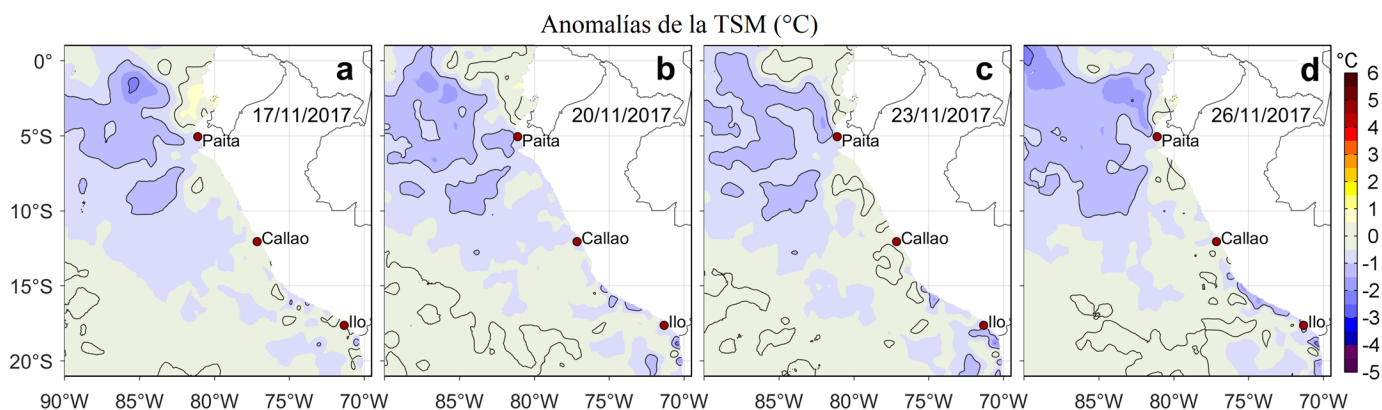
Figura 3. Anomalías de la Temperatura Superficial del Mar (°C) para los días: a) 17, b) 20, c) 23, y d) 26 de noviembre de 2017. Las anomalías se calcularon respecto de la climatología para el periodo 2007-2016. Datos: OSTIA-UKMO-L4-GLOB-v2.0 (UK Met Office, 2012; Donlon et al, 2012). Procesamiento: LHF/AFIOF/DGIOCC/IMARPE.
