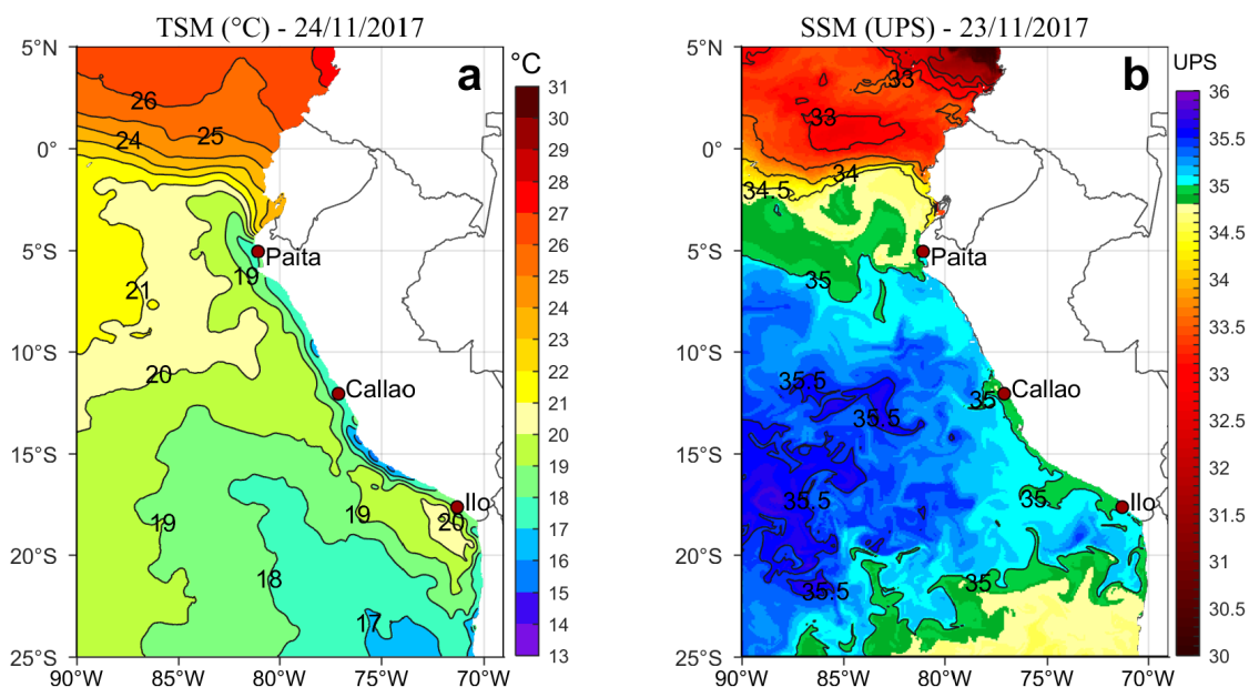
Figura 2. a) Temperatura superficial del mar (°C) y b) Salinidad superficial del mar (UPS) para el 24 y 23 de noviembre, respectivamente. Datos: OSTIA-UKMO-L4-GLOB-v2.0 (UK Met Office, 2012; Donlon et al, 2012) disponible en https://podaac.jpl.nasa.gov/dataset/OSTIA-UKMO-L4-GLOB-v2.0 para (a) y Hybrid Coordinate Ocean Model (HYCOM; Halliwell et al., 1998; 2000; Bleck, 2001) para (b). Procesamiento: LHF/AFIOF/DGIOCC/IMARPE.
