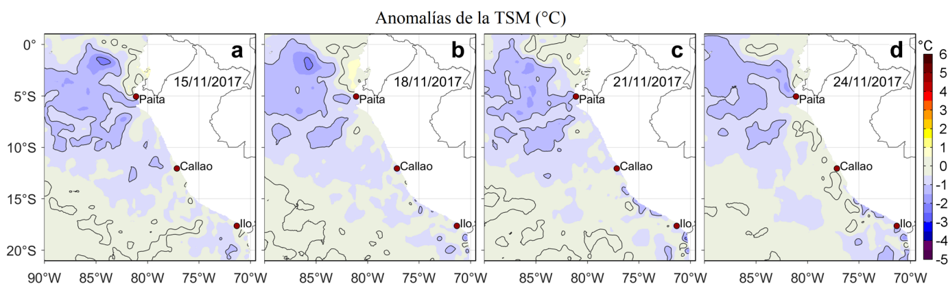
Figura 3. Anomalías de la Temperatura Superficial del Mar (°C) para los días: a) 15, b) 18, c) 21, y d) 24 de noviembre de 2017. Las anomalías se calcularon respecto de la climatología para el periodo 2007-2016. Datos: OSTIA-UKMO-L4-GLOB-v2.0 (UK Met Office, 2012; Donlon et al, 2012). Procesamiento: LHF/AFIOF/DGIOCC/IMARPE.
