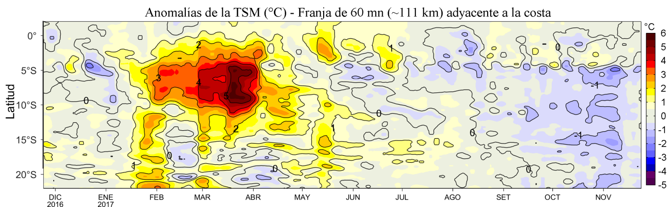
Figura 4. Variación promedio de las anomalías de la temperatura superficial del mar (°C) para una franja de 60 mn (~111 km) adyacente al litoral peruano para los últimos doce meses al 24 de noviembre de 2017. Datos: OSTIA-UKMO-L4-GLOB-v2.0 (UK Met. Office, 2012; Donlon et al, 2012) disponible en https://podaac.jpl.nasa.gov/dataset/OSTIA-UKMO-L4-GLOB-v2.0 . Las anomalías se calcularon con respecto al periodo 2007-2016. Procesamiento: LHF/AFIOF/DGIOCC/IMARPE.
