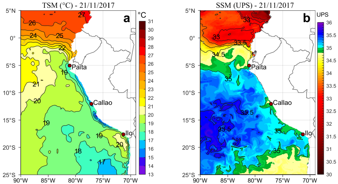
Figura 2. a) Temperatura superficial del mar (°C) y b) Salinidad superficial del mar (UPS) para el 21 de noviembre. Datos: OSTIA-UKMO-L4-GLOB-v2.0 (UK Met Office, 2012; Donlon et al, 2012) disponible en https://podaac.jpl.nasa.gov/dataset/OSTIA-UKMO-L4-GLOB-v2.0 para (a) y Hybrid Coordinate Ocean Model (HYCOM; Halliwell et al., 1998; 2000; Bleck, 2001) para (b). Procesamiento: LHF/AFIOF/DGIOCC/IMARPE.
