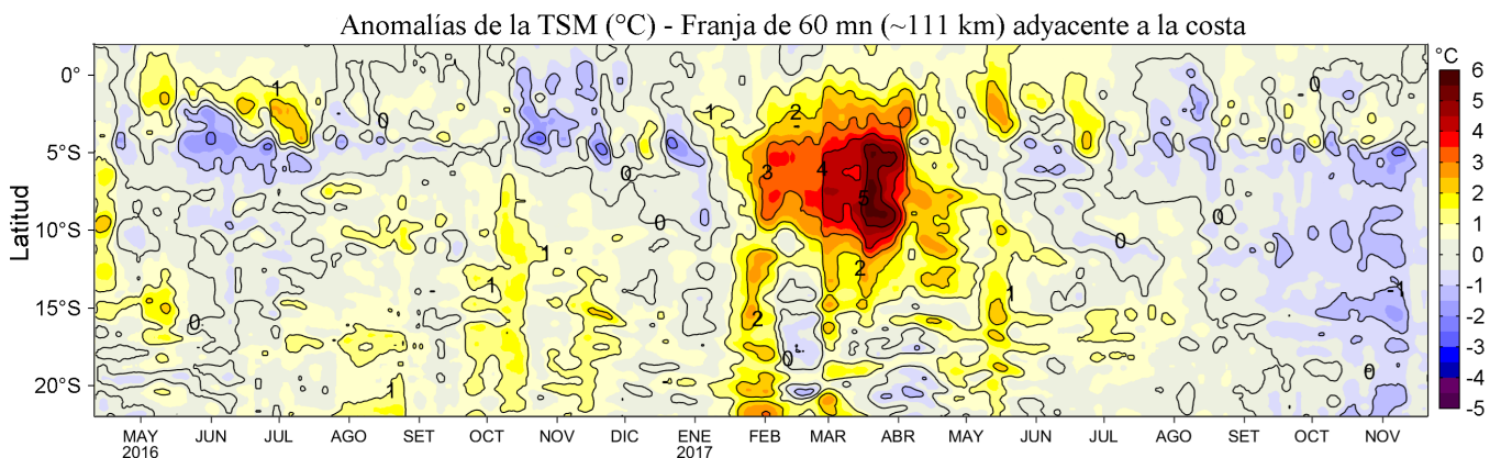
Figura 4. Variación promedio de las anomalías de la temperatura superficial del mar (°C) para una franja de 60 mn (~111 km) adyacente al litoral peruano para los últimos doce meses al 21 de noviembre de 2017. Datos: OSTIA-UKMO-L4-GLOB-v2.0 (UK Met. Office, 2012; Donlon et al, 2012) disponible en https://podaac.jpl.nasa.gov/dataset/OSTIA-UKMO-L4-GLOB-v2.0 . Las anomalías se calcularon con respecto al periodo 2007-2016. Procesamiento: LHF/AFIOF/DGIOCC/IMARPE.
