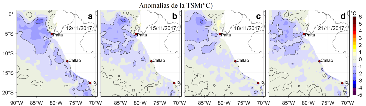
Figura 3. Anomalías de la Temperatura Superficial del Mar (°C) para los días: a) 12, b) 15, c) 18, y d) 21 de noviembre de 2017. Las anomalías se calcularon respecto de la climatología para el periodo 2007-2016. Datos: OSTIA-UKMO-L4-GLOB-v2.0 (UK Met Office, 2012; Donlon et al, 2012). Procesamiento: LHF/AFIOF/DGIOCC/IMARPE.
