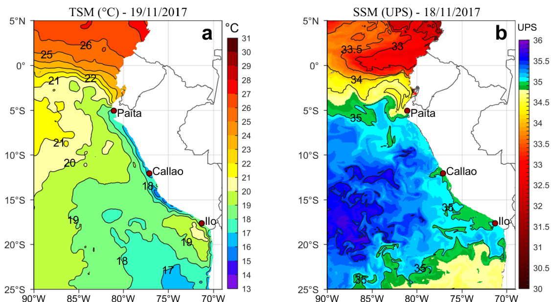
Figura 2. a) Temperatura superficial del mar (°C) y b) Salinidad superficial del mar (UPS) para el 19 y 18 de noviembre, respectivamente. Datos: OSTIA-UKMO-L4-GLOB-v2.0 (UK Met Office, 2012; Donlon et al, 2012) disponible en https://podaac.jpl.nasa.gov/dataset/OSTIA-UKMO-L4-GLOB-v2.0 para (a) y Hybrid Coordinate Ocean Model (HYCOM; Halliwell et al., 1998; 2000; Bleck, 2001)
