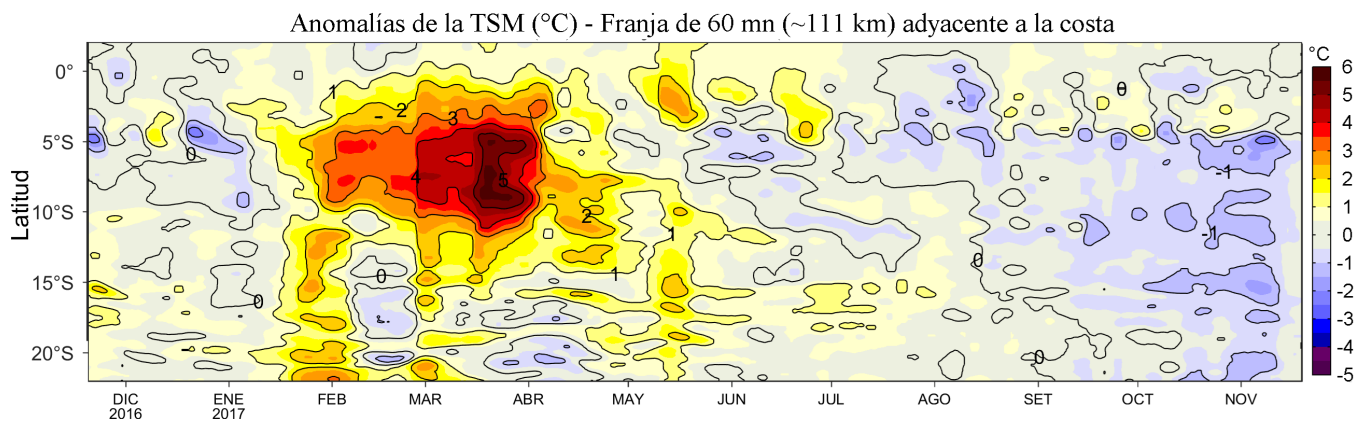
Figura 4. Variación promedio de las anomalías de la temperatura superficial del mar (°C) para una franja de 60 mn (~111 km) adyacente a la costa para los últimos doce meses al 19 de noviembre de 2017. Datos: OSTIA-UKMO-L4-GLOB-v2.0 (UK Met. Office, 2012; Donlon et al, 2012) disponible en https://podaac.jpl.nasa.gov/dataset/OSTIA-UKMO-L4-GLOB-v2.0 . Las anomalías se calcularon con respecto al periodo 2007-2016. Procesamiento: LHF/AFIOF/DGIOCC/IMARPE.
