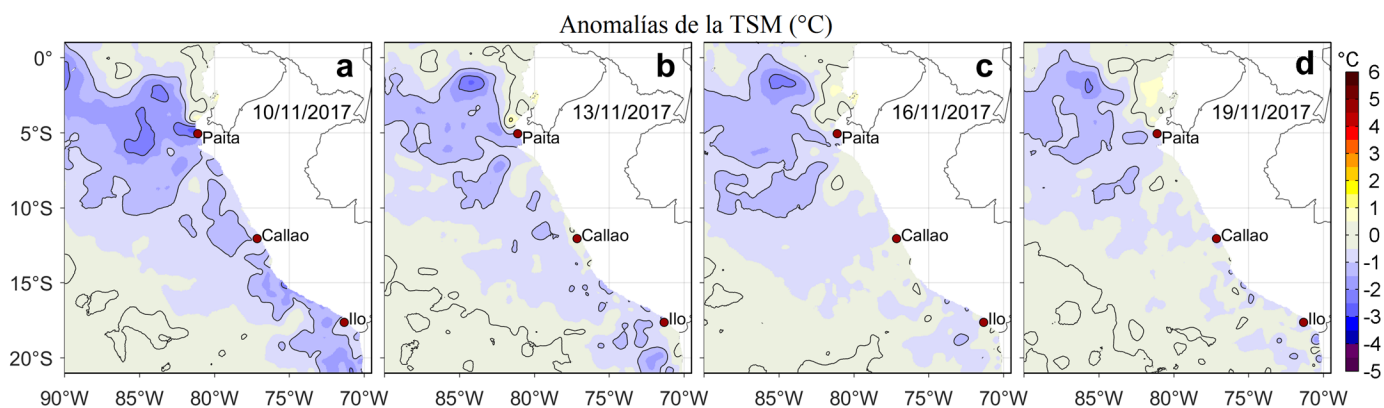
Figura 3. Anomalías de la Temperatura Superficial del Mar (°C) para los días: a) 10, b) 13, c) 16, y d) 19 de noviembre de 2017. Las anomalías se calcularon respecto de la climatología para el periodo 2007-2016. Datos: OSTIA-UKMO-L4-GLOB-v2.0 (UK Met Office, 2012; Donlon et al, 2012). Procesamiento: LHF/AFIOF/DGIOCC/IMARPE.
