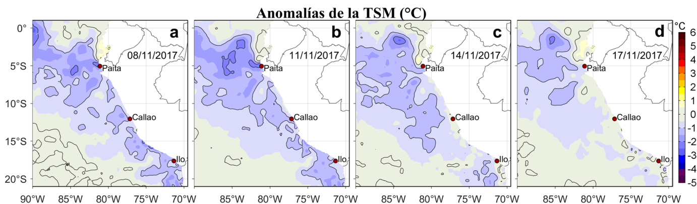
Figura 3. Anomalías de la Temperatura Superficial del Mar (°C) para los días: a) 08, b) 11, c) 14, y d) 17 de noviembre de 2017. Las anomalías se calcularon respecto de la climatología para el periodo 2007-2016. Datos: OSTIA-UKMO-L4-GLOB-v2.0 (UK Met Office, 2012; Donlon et al, 2012). Procesamiento: LHF/AFIOF/DGIOCC/IMARPE.
