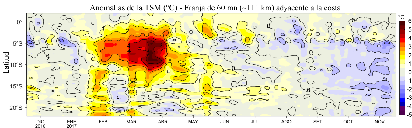
Figura 4. Variación promedio de las anomalías de la temperatura superficial del mar (°C) para una franja de 60 mn (~111 km) adyacente al litoral peruano para los últimos doce meses al 17 de noviembre de 2017. Datos: OSTIA-UKMO-L4-GLOB-v2.0 (UK Met. Office, 2012; Donlon et al, 2012) disponible en https://podaac.jpl.nasa.gov/dataset/OSTIA-UKMO-L4-GLOB-v2.0 . Las anomalías se calcularon con respecto al periodo 2007-2016. Procesamiento: LHF/AFIOF/DGIOCC/IMARPE.
