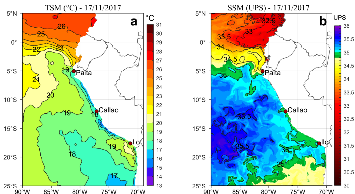
Figura 2. a) Temperatura superficial del mar (°C) y b) Salinidad superficial del mar (UPS) para el 17 de noviembre respectivamente. Datos: OSTIA-UKMO-L4-GLOB-v2.0 (UK Met Office, 2012; Donlon et al, 2012) disponible en https://podaac.jpl.nasa.gov/dataset/OSTIA-UKMO-L4-GLOB-v2.0 para (a) y Hybrid Coordinate Ocean Model (HYCOM; Halliwell et al., 1998; 2000; Bleck, 2001) para (b). Procesamiento: LHF/AFIOF/DGIOCC/IMARPE.
