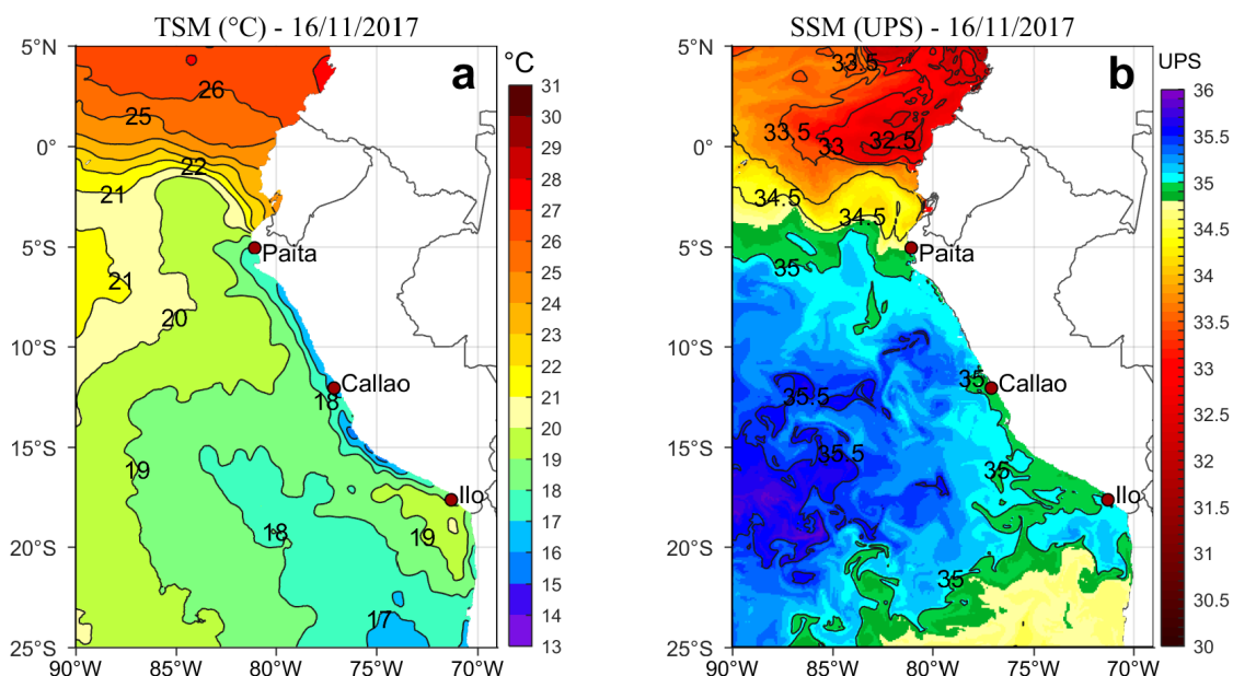
Figura 2. a) Temperatura superficial del mar (°C) y b) Salinidad superficial del mar (UPS) para el 16 de noviembre respectivamente. Datos: OSTIA-UKMO-L4-GLOB-v2.0 (UK Met Office, 2012; Donlon et al, 2012) disponible en https://podaac.jpl.nasa.gov/dataset/OSTIA-UKMO-L4-GLOB-v2.0 para (a) y Hybrid Coordinate Ocean Model (HYCOM; Halliwell et al., 1998; 2000; Bleck, 2001) para (b). Procesamiento: LHF/AFIOF/DGIOCC/IMARPE.
