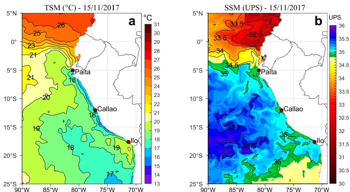
Figura 2. a) Temperatura superficial del mar (°C) y b) Salinidad superficial del mar (UPS) para el 15 de noviembre respectivamente. Datos: OSTIA-UKMO-L4-GLOB-v2.0 (UK Met Office, 2012; Donlon et al, 2012) disponible en https://podaac.jpl.nasa.gov/dataset/OSTIA-UKMO-L4-GLOB-v2.0 para (a) y Hybrid Coordinate Ocean Model (HYCOM; Halliwell et al., 1998; 2000; Bleck, 2001) para (b). Procesamiento: LHF/AFIOF/DGIOCC/IMARPE.
