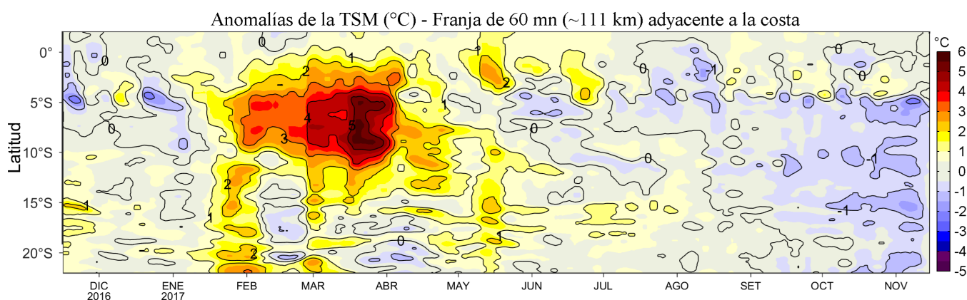
Figura 4. Variación promedio de las anomalías de la temperatura superficial del mar (°C) para una franja de 60 mn (~111 km) adyacente al litoral peruano para los últimos doce meses al 15 de noviembre de 2017. Datos: OSTIA-UKMO-L4-GLOB-v2.0 (UK Met. Office, 2012; Donlon et al, 2012) disponible en https://podaac.jpl.nasa.gov/dataset/OSTIA-UKMO-L4-GLOB-v2.0 . Las anomalías se calcularon con respecto al periodo 2007-2016. Procesamiento: LHF/AFIOF/DGIOCC/IMARPE.
