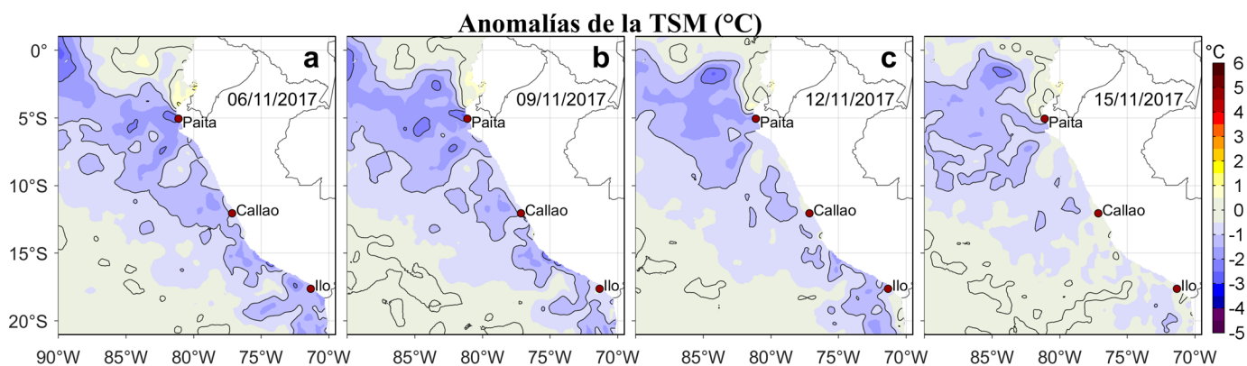
Figura 3. Anomalías de la Temperatura Superficial del Mar (°C) para los días: a) 06, b) 09, c) 12, y d) 15 de noviembre de 2017. Las anomalías se calcularon respecto de la climatología para el periodo 2007-2016. Datos: OSTIA-UKMO-L4-GLOB-v2.0 (UK Met Office, 2012; Donlon et al, 2012). Procesamiento: LHF/AFIOF/DGIOCC/IMARPE.
