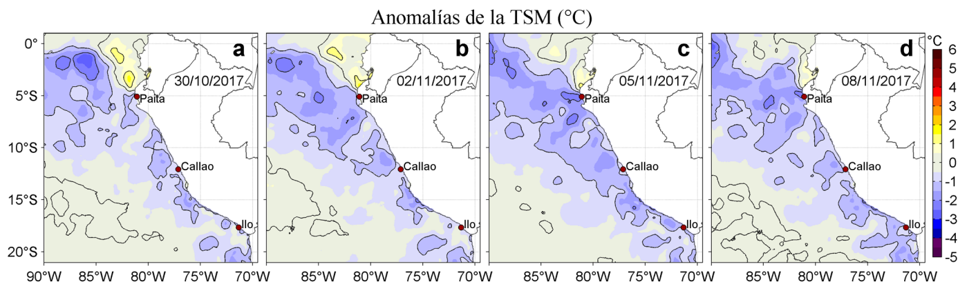
Figura 3. Anomalías de la Temperatura Superficial del Mar ( ^{\circ}\text{C} ) para los días: a) 30, de octubre, y b) 02, c) 05, y d) 08 de noviembre de 2017. Las anomalías se calcularon respecto de la climatología para el periodo 2007-2016. Datos: OSTIA-UKMO-L4-GLOB-v2.0 (UK Met Office, 2012; Donlon et al, 2012). Procesamiento: LHF/AFIOF/DGIOCC/IMARPE.
