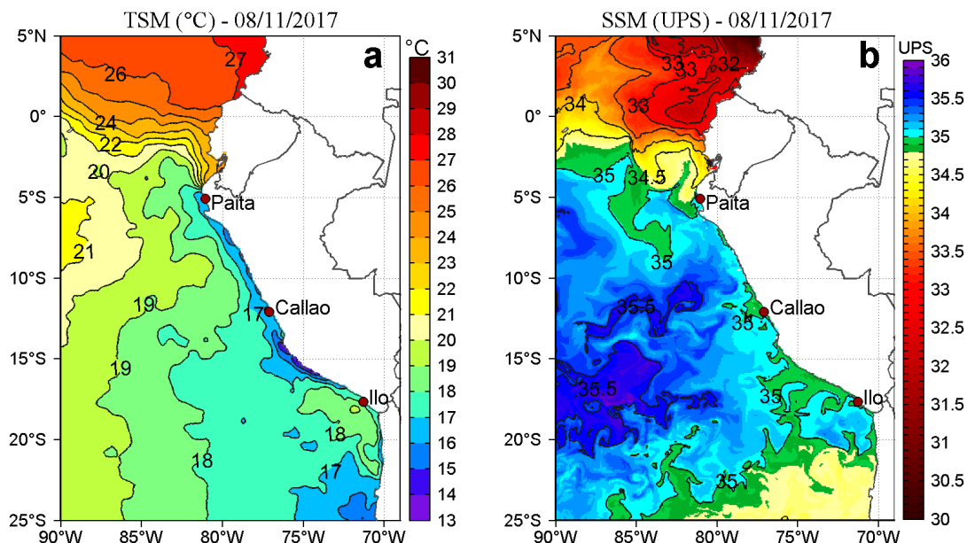
Figura 2. a) Temperatura superficial del mar ( ^{\circ}\text{C} ) y b) Salinidad superficial del mar (UPS) para el 08 de noviembre respectivamente. Datos: OSTIA-UKMO-L4-GLOB-v2.0 (UK Met Office, 2012; Donlon et al, 2012) disponible en https://podaac.jpl.nasa.gov/dataset/OSTIA-UKMO-L4-GLOB-v2.0 para (a) y Hybrid Coordinate Ocean Model (HYCOM; Halliwell et al., 1998; 2000; Bleck, 2001) para (b). Procesamiento: LHF/AFIOF/DGIOCC/IMARPE.
