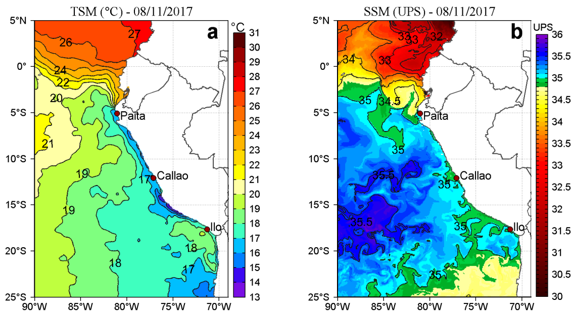
Figura 2. a) Temperatura superficial del mar (°C) y b) Salinidad superficial del mar (UPS) para el 08 de noviembre respectivamente. Datos: OSTIA-UKMO-L4-GLOB-v2.0 (UK Met Office, 2012; Donlon et al, 2012) disponible en https://podaac.jpl.nasa.gov/dataset/OSTIA-UKMO-L4-GLOB-v2.0 para (a) y Hybrid Coordinate Ocean Model (HYCOM; Halliwell et al., 1998; 2000; Bleck, 2001) para (b). Procesamiento: LHF/AFIOF/DGIOCC/IMARPE.
