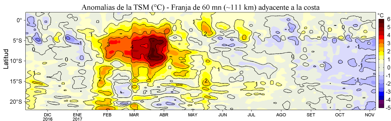
Figura 4. Variación promedio de las anomalías de la temperatura superficial del mar (°C) para una franja de 60 mn (~111 km) adyacente al litoral peruano para los últimos doce meses al 08 de noviembre de 2017. Datos: OSTIA-UKMO-L4-GLOB-v2.0 (UK Met. Office, 2012; Donlon et al, 2012) disponible en https://podaac.jpl.nasa.gov/dataset/OSTIA-UKMO-L4-GLOB-v2.0 . Las anomalías se calcularon con respecto al periodo 2007-2016. Procesamiento: LHF/AFIOF/DGIOCC/IMARPE.
