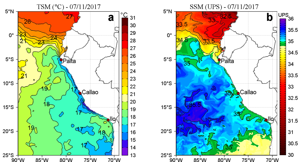
Figura 2. a) Temperatura superficial del mar (°C) y b) Salinidad superficial del mar (UPS) para el 07 de noviembre respectivamente. Datos: OSTIA-UKMO-L4-GLOB-v2.0 (UK Met Office, 2012; Donlon et al, 2012) disponible en https://podaac.jpl.nasa.gov/dataset/OSTIA-UKMO-L4-GLOB-v2.0 para (a) y Hybrid Coordinate Ocean Model (HYCOM; Halliwell et al., 1998; 2000; Bleck, 2001) para (b). Procesamiento: LHF/AFIOF/DGIOCC/IMARPE.
