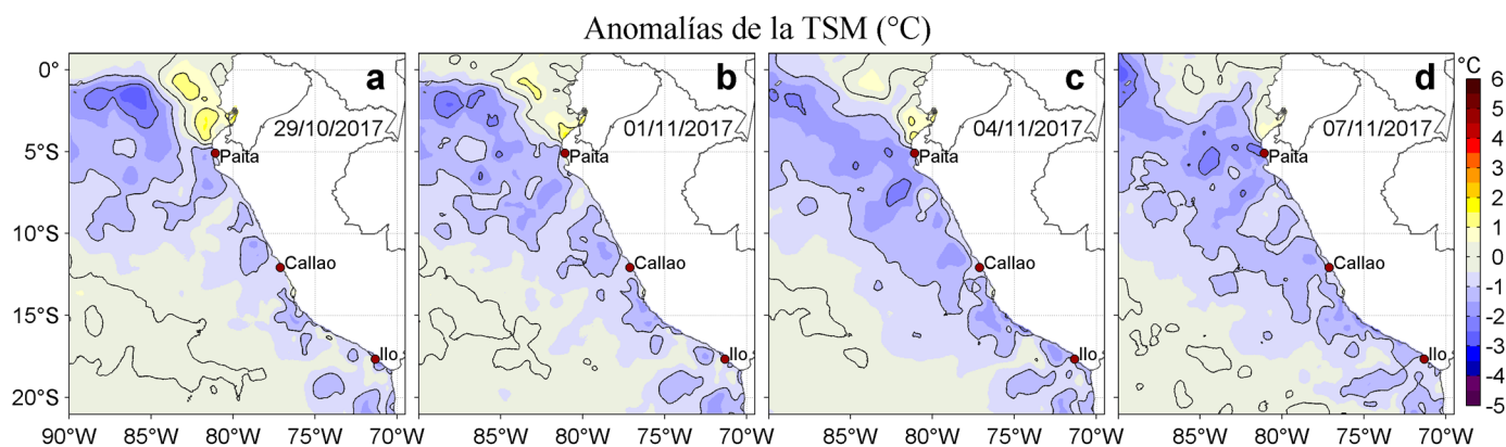
Figura 3. Anomalías de la Temperatura Superficial del Mar (°C) para los días: a) 29, de noviembre, y b) 01 c) 04, y d) 07 de noviembre de 2017. Las anomalías se calcularon respecto de la climatología para el periodo 2007-2016. Datos: OSTIA-UKMO-L4-GLOB-v2.0 (UK Met Office, 2012; Donlon et al, 2012). Procesamiento: LHF/AFIOF/DGIOCC/IMARPE.
