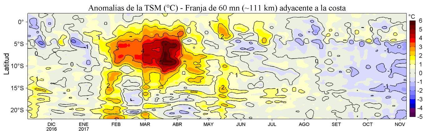
Figura 4. Variación promedio de las anomalías de la temperatura superficial del mar (°C) para una franja de 60 mn (~111 km) adyacente al litoral peruano para los últimos doce meses al 07 de noviembre de 2017. Datos: OSTIA-UKMO-L4-GLOB-v2.0 (UK Met. Office, 2012; Donlon et al, 2012) disponible en https://podaac.jpl.nasa.gov/dataset/OSTIA-UKMO-L4-GLOB-v2.0 . Las anomalías se calcularon con respecto al periodo 2007-2016. Procesamiento: LHF/AFIOF/DGIOCC/IMARPE.
