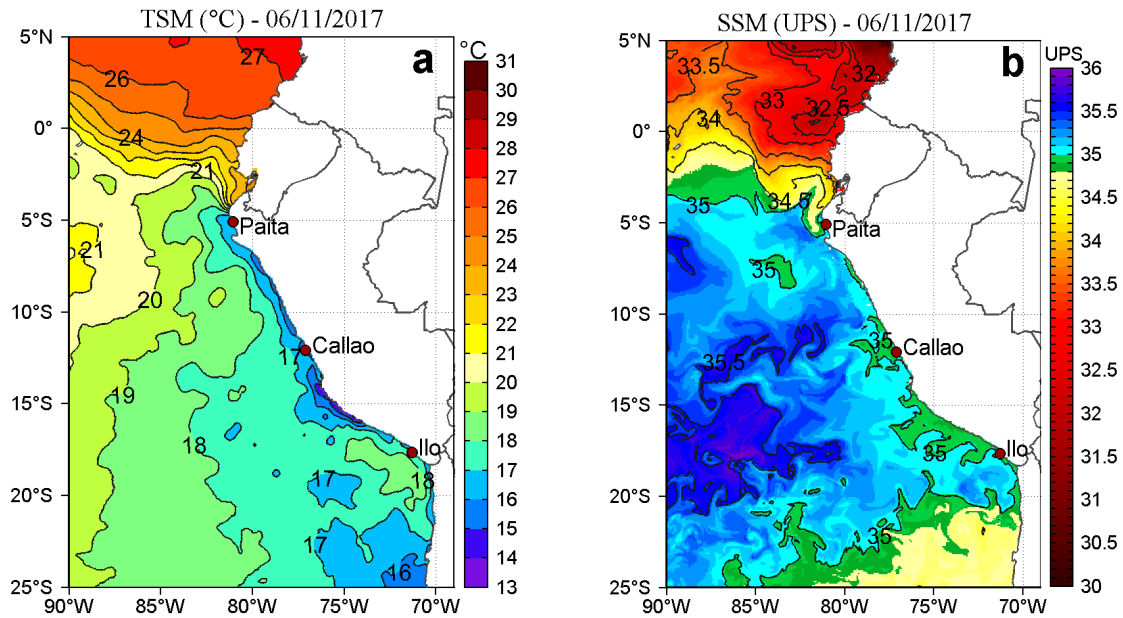
Figura 2. a) Temperatura superficial del mar ( ^{\circ}\text{C} ) y b) Salinidad superficial del mar (UPS) para el 06 de noviembre. Datos: OSTIA-UKMO-L4-GLOB-v2.0 (UK Met Office, 2012; Donlon et al, 2012) disponible en https://podaac.jpl.nasa.gov/dataset/OSTIA-UKMO-L4-GLOB-v2.0 para (a) y Hybrid Coordinate Ocean Model (HYCOM; Halliwell et al., 1998; 2000; Bleck, 2001) para (b). Procesamiento: LHF/AFIOF/DGIOCC/IMARPE.
