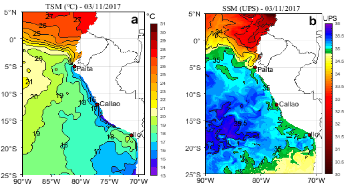
Figura 2. a) Temperatura superficial del mar (°C) y b) Salinidad superficial del mar (UPS) actualizado al 03 de noviembre: OSTIA-UKMO-L4-GLOB-v2.0 (UK Met Office, 2012; Donlon et al, 2012) disponible en https://podaac.jpl.nasa.gov/dataset/OSTIA-UKMO-L4-GLOB-v2.0 para (a) y Hybrid Coordinate Ocean Model (HYCOM; Halliwell et al., 1998; 2000; Bleck, 2001) para (b). Procesamiento: LHF/AFIOF/DGIOCC/IMARPE.
