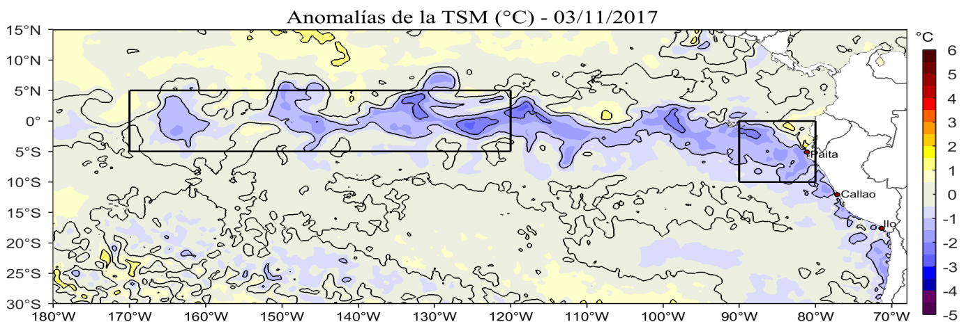
Figura 1. Anomalías de la temperatura superficial del mar ( ^\circ\text{C} ) en el océano Pacífico tropical. Las regiones Niño 3.4 ( 5^\circ\text{N} - 5^\circ\text{S} , 170^\circ\text{W} - 120^\circ\text{W} ) y Niño 1+2 ( 0^\circ - 10^\circ\text{S} , 90^\circ\text{W} - 80^\circ\text{W} ) en los sectores central y oriental del océano, respectivamente, están delimitadas con una línea de color negro. Climatología: 2007-2016. Datos: OSTIA-UKMO-L4-GLOB-v2.0 (UK Met Office, 2012; Donlon et al, 2012) disponible en https://podaac.jpl.nasa.gov/dataset/OSTIA-UKMO-L4-GLOB-v2.0 . Procesamiento: IMARPE.
