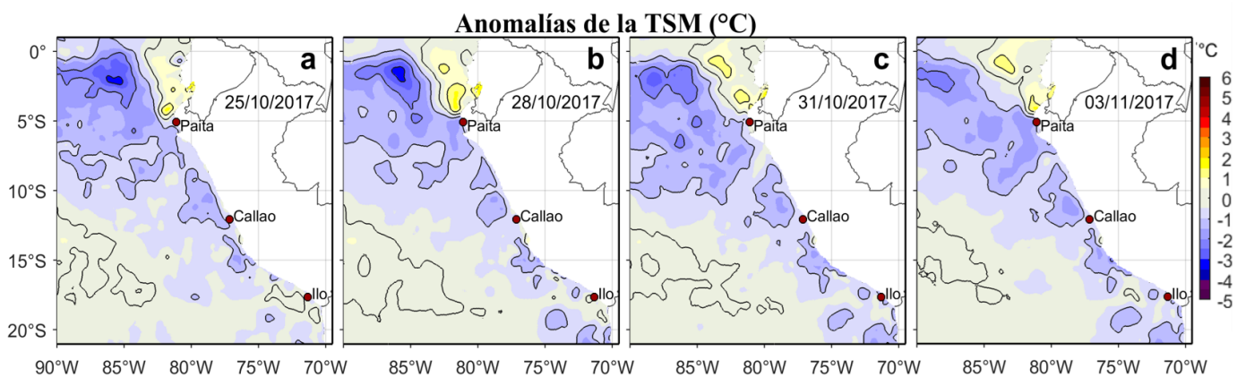
Figura 3. Anomalías de la Temperatura Superficial del Mar (°C) para los días: a) 25, b) 28, c) 31 de octubre y d) 03 de noviembre de 2017. Las anomalías se calcularon respecto de la climatología para el periodo 2007-2016. Datos: OSTIA-UKMO-L4-GLOB-v2.0 (UK Met Office, 2012; Donlon et al, 2012). Procesamiento: LHF/AFIOF/DGIOCC/IMARPE.
