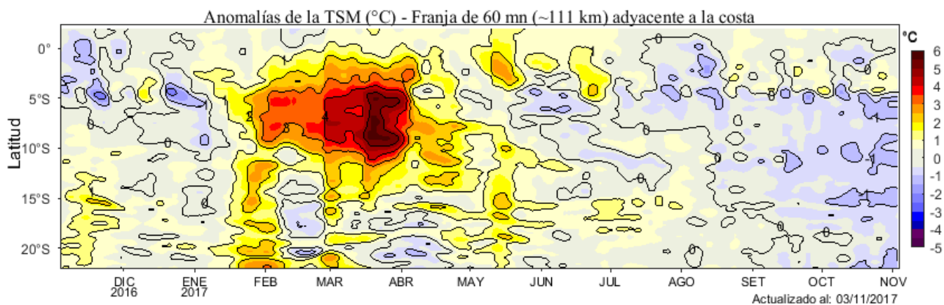
Figura 4. Variación promedio de las anomalías de la temperatura superficial del mar (°C) para una franja de 60 mn (~111 km) adyacente a la costa al litoral peruano para los últimos doce meses al 03 de noviembre del 2017. Datos: OSTIA-UKMO-L4-GLOB-v2.0 (UK Met. Office, 2012; Donlon et al, 2012) disponible en https://podaac.jpl.nasa.gov/dataset/OSTIA-UKMO-L4-GLOB-v2.0 . Las anomalías se calcularon con respecto al periodo 2007-2016. Procesamiento: LHF/AFIOF/DGIOCC/IMARPE.
