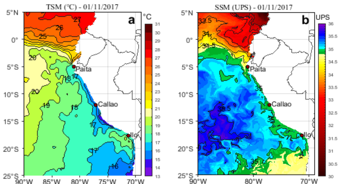
Figura 2. a) Temperatura superficial del mar (°C) y b) Salinidad superficial del mar (UPS) actualizado al 01 de noviembre: OSTIA-UKMO-L4-GLOB-v2.0 (UK Met Office, 2012; Donlon et al, 2012) disponible en https://podaac.jpl.nasa.gov/dataset/OSTIA-UKMO-L4-GLOB-v2.0 para (a) y Hybrid Coordinate Ocean Model (HYCOM; Halliwell et al., 1998; 2000; Bleck, 2001) para (b). Procesamiento: LHF/AFIOF/DGIOCC/IMARPE.
