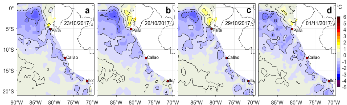
Figura 3. Anomalías de la Temperatura Superficial del Mar (°C) para los días: a) 23, b) 26, c) 29 de octubre y d) 01 de noviembre del 2017. Las anomalías se calcularon respecto de la climatología para el periodo 2007-2016. Datos: OSTIA-UKMO-L4-GLOB-v2.0 (UK Met Office, 2012; Donlon et al, 2012). Procesamiento: LHF/AFIOF/DGIOCC/IMARPE.
