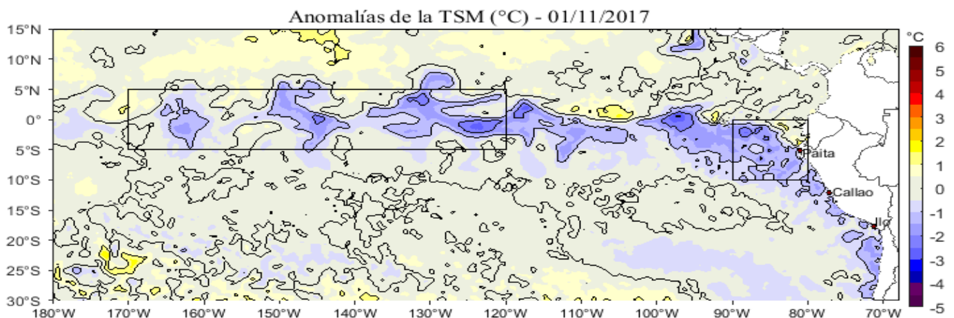
Figura 1. Anomalías de la temperatura superficial del mar (°C) en el océano Pacífico tropical. Las regiones Niño 3.4 (5°N-5°S, 170°W-120°W) y Niño 1+2 (0°-10°S, 90°W-80°W) en los sectores central y oriental del océano, respectivamente, están delimitadas con una línea de color negro. Climatología: 2007-2016. Datos: OSTIA-UKMO-L4-GLOB-v2.0 (UK Met Office, 2012; Donlon et al, 2012) disponible en https://podaac.jpl.nasa.gov/dataset/OSTIA-UKMO-L4-GLOB-v2.0 . Procesamiento: IMARPE.
