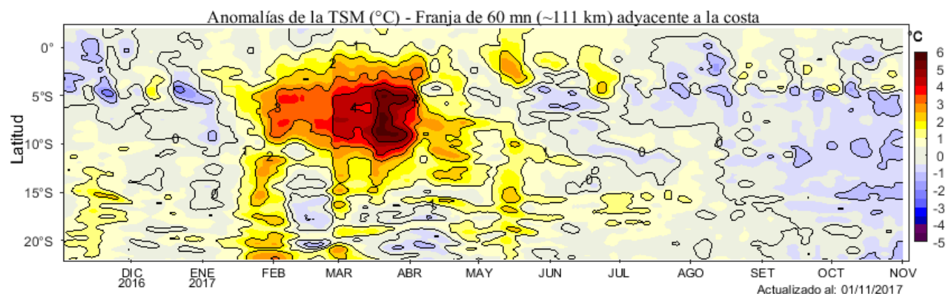
Figura 4. Variación promedio de las anomalías de la temperatura superficial del mar (°C) para una franja de 60 mn (~111 km) adyacente al litoral peruano para los últimos doce meses al 01 de noviembre del 2017. Datos: OSTIA-UKMO-L4-GLOB-v2.0 (UK Met. Office, 2012; Donlon et al, 2012) disponible en https://podaac.jpl.nasa.gov/dataset/OSTIA-UKMO-L4-GLOB-v2.0 . Las anomalías se calcularon con respecto al periodo 2007-2016. Procesamiento: LHF/AFIOF/DGIOCC/IMARPE.
