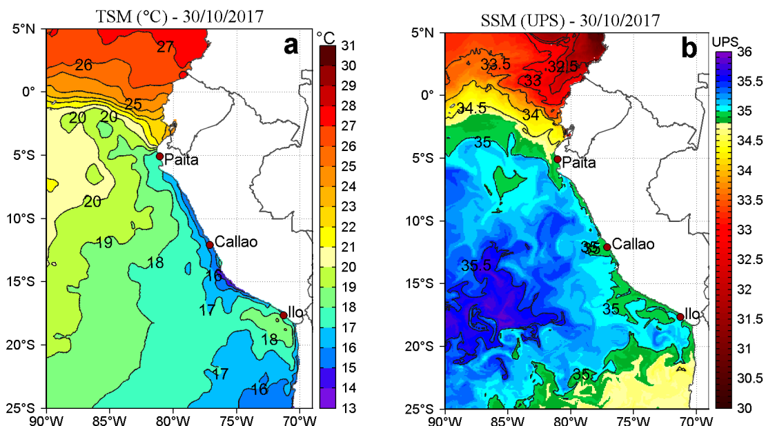
Figura 2. a) Temperatura superficial del mar (°C) y b) Salinidad superficial del mar (UPS) para el 30 de octubre: OSTIA-UKMO-L4-GLOB-v2.0 (UK Met Office, 2012; Donlon et al, 2012) disponible en https://podaac.jpl.nasa.gov/dataset/OSTIA-UKMO-L4-GLOB-v2.0 para (a) y Hybrid Coordinate Ocean Model (HYCOM; Halliwell et al., 1998; 2000; Bleck, 2001) para (b). Procesamiento: LHF/AFIOF/DGIOCC/IMARPE.
