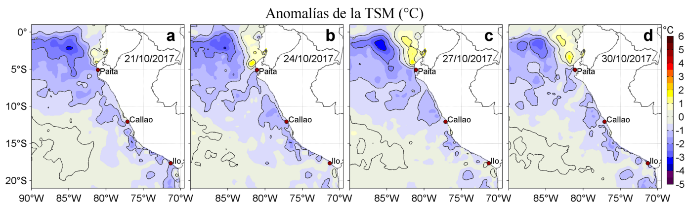
Figura 3. Anomalías de la Temperatura Superficial del Mar (°C) para los días: a) 21, b) 24, c) 27, y d) 30 de octubre de 2017. Las anomalías se calcularon respecto de la climatología para el periodo 2007-2016. Datos: OSTIA-UKMO-L4-GLOB-v2.0 (UK Met Office, 2012; Donlon et al, 2012). Procesamiento: LHF/AFIOF/DGIOCC/IMARPE.
