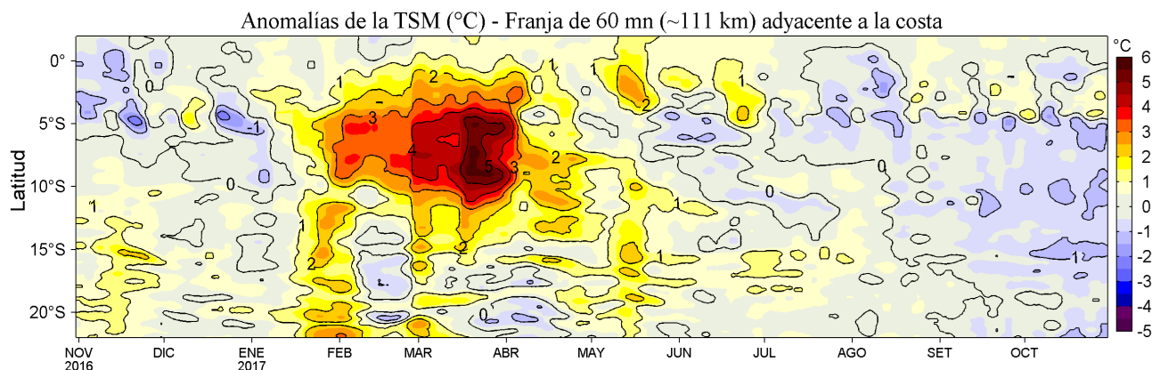
Figura 4. Variación promedio de las anomalías de la temperatura superficial del mar (°C) para una franja de 60 mn (~111 km) adyacente al litoral peruano para los últimos doce meses al 30 de octubre de 2017. Datos: OSTIA-UKMO-L4-GLOB-v2.0 (UK Met. Office, 2012; Donlon et al, 2012) disponible en https://podaac.jpl.nasa.gov/dataset/OSTIA-UKMO-L4-GLOB-v2.0 . Las anomalías se calcularon con respecto al periodo 2007-2016. Procesamiento: LHF/AFIOF/DGIOCC/IMARPE.
