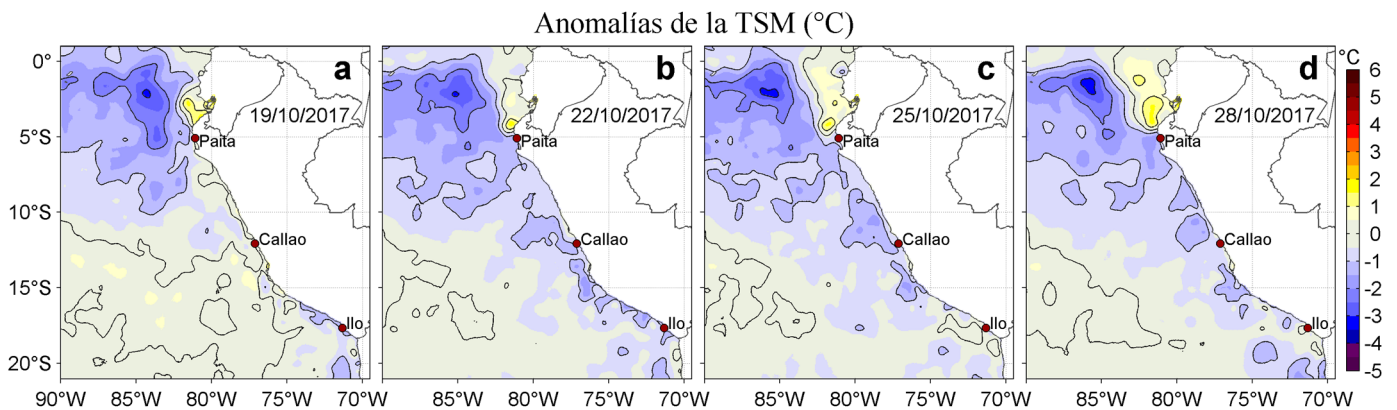
Figura 3. Anomalías de la Temperatura Superficial del Mar (°C) para los días: a) 19, b) 22, c) 25, y d) 28 de octubre de 2017. Las anomalías se calcularon respecto de la climatología para el periodo 2007-2016. Datos: OSTIA-UKMO-L4-GLOB-v2.0 (UK Met Office, 2012; Donlon et al, 2012). Procesamiento: LHF/AFIOF/DGIOCC/IMARPE.
