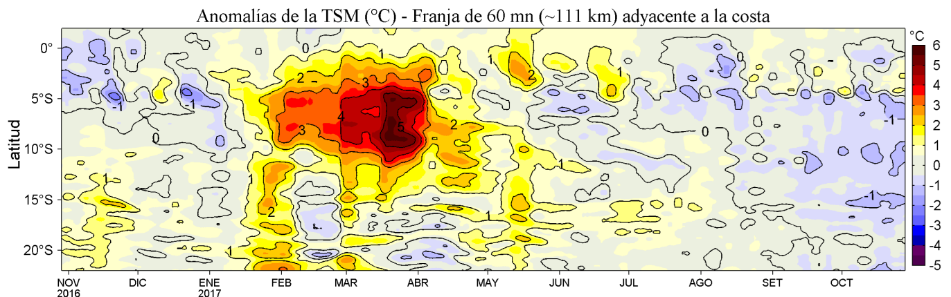
Figura 4. Variación promedio de las anomalías de la temperatura superficial del mar (°C) para una franja de 60 mn (~111 km) adyacente al litoral peruano para los últimos doce meses al 28 de octubre de 2017. Datos: OSTIA-UKMO-L4-GLOB-v2.0 (UK Met. Office, 2012; Donlon et al, 2012) disponible en https://podaac.jpl.nasa.gov/dataset/OSTIA-UKMO-L4-GLOB-v2.0 . Las anomalías se calcularon con respecto al periodo 2007-2016. Procesamiento: LHF/AFIOF/DGIOCC/IMARPE.
