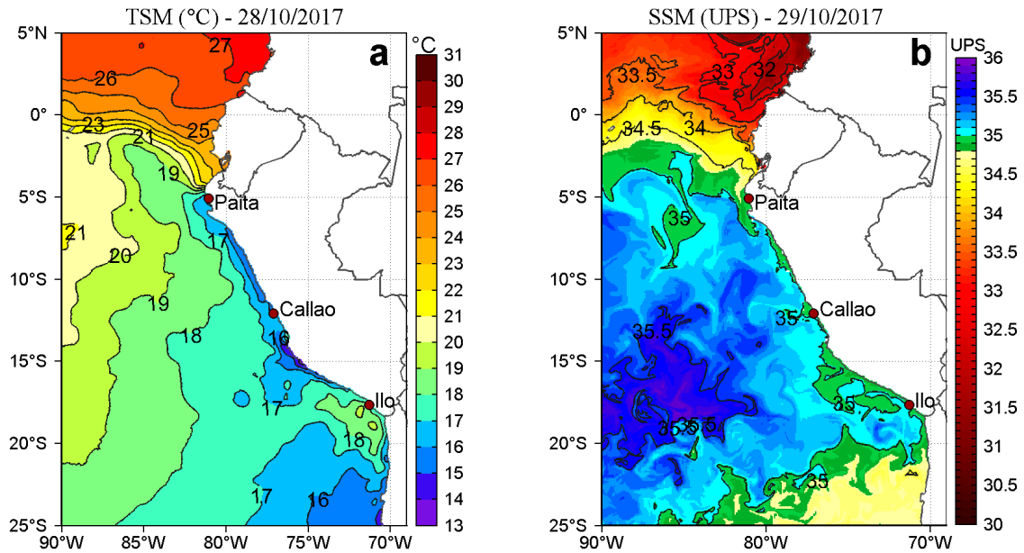
Figura 2. a) Temperatura superficial del mar (°C) y b) Salinidad superficial del mar (UPS) para el 28 y 29 de octubre, respectivamente. Datos: OSTIA-UKMO-L4-GLOB-v2.0 (UK Met Office, 2012; Donlon et al, 2012) disponible en https://podaac.jpl.nasa.gov/dataset/OSTIA-UKMO-L4-GLOB-v2.0 para (a) y Hybrid Coordinate Ocean Model (HYCOM; Halliwell et al., 1998; 2000; Bleck, 2001) para (b). Procesamiento: LHF/AFIOF/DGIOCC/IMARPE.
