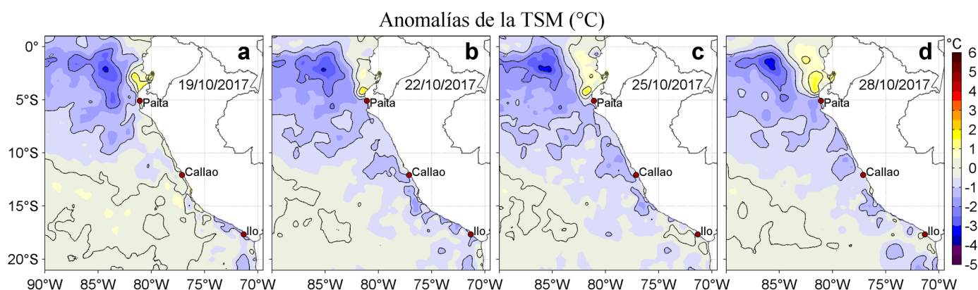
Figura 3. Anomalías de la Temperatura Superficial del Mar ( ^{\circ}\text{C} ) para los días: a) 19, b) 22, c) 25, y d) 28 de octubre de 2017. Las anomalías se calcularon respecto de la climatología para el periodo 2007-2016. Datos: OSTIA-UKMO-L4-GLOB-v2.0 (UK Met Office, 2012; Donlon et al, 2012). Procesamiento: LHF/AFIOF/DGIOCC/IMARPE.
