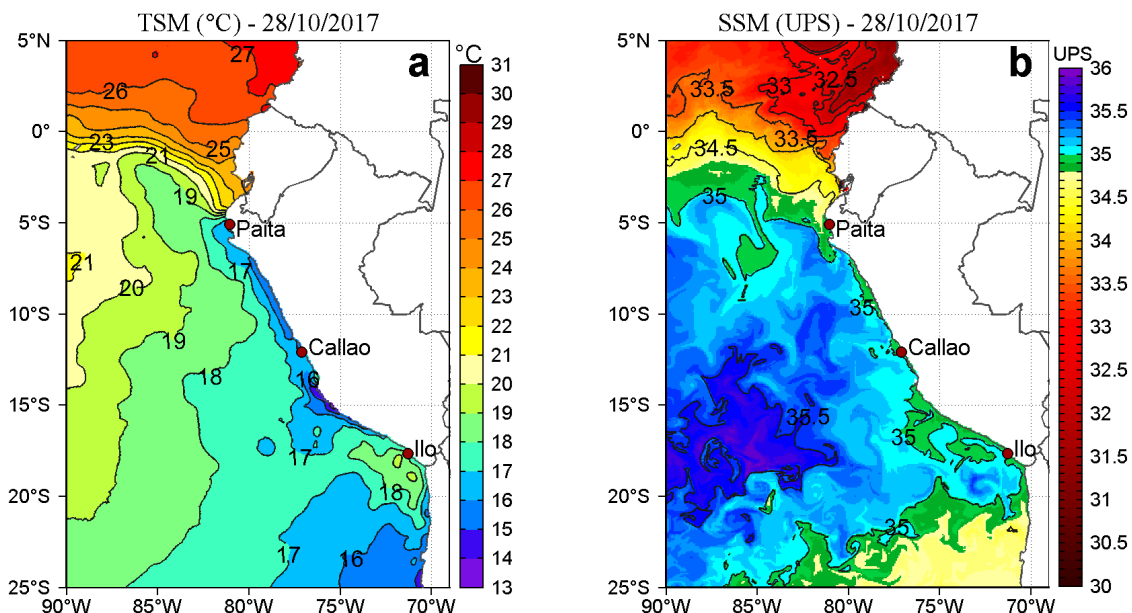
Figura 2. a) Temperatura superficial del mar ( ^{\circ}\text{C} ) y b) Salinidad superficial del mar (UPS) para el 28 de octubre. Datos: OSTIA-UKMO-L4-GLOB-v2.0 (UK Met Office, 2012; Donlon et al, 2012) disponible en https://podaac.jpl.nasa.gov/dataset/OSTIA-UKMO-L4-GLOB-v2.0 para (a) y Hybrid Coordinate Ocean Model (HYCOM; Halliwell et al., 1998; 2000; Bleck, 2001) para (b). Procesamiento: LHF/AFIOF/DGIOCC/IMARPE.
