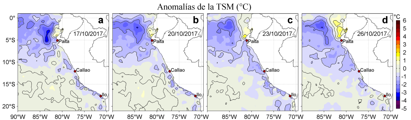
Figura 3. Anomalías de la Temperatura Superficial del Mar ( ^{\circ}\text{C} ) para los días: a) 17, b) 20, c) 23, y d) 26 de octubre de 2017. Las anomalías se calcularon respecto de la climatología para el periodo 2007-2016. Datos: OSTIA-UKMO-L4-GLOB-v2.0 (UK Met Office, 2012; Donlon et al., 2012). Procesamiento: LHF/AFIOF/DGIOCC/IMARPE.
