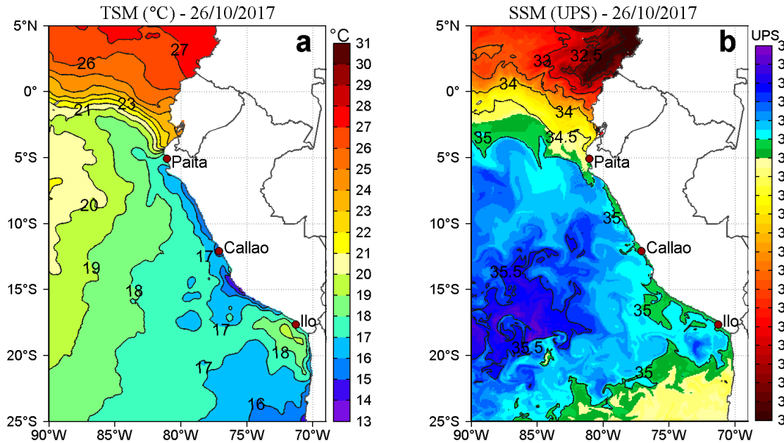
Figura 2. a) Temperatura superficial del mar ( ^{\circ}\text{C} ) y b) Salinidad superficial del mar (UPS) para el 26 de octubre. Datos: OSTIA-UKMO-L4-GLOB-v2.0 (UK Met Office, 2012; Donlon et al., 2012) disponible en https://podaac.jpl.nasa.gov/dataset/OSTIA-UKMO-L4-GLOB-v2.0 para (a) y Hybrid Coordinate Ocean Model (HYCOM; Halliwell et al., 1998; 2000; Bleck, 2001) para (b). Procesamiento: LHF/AFIOF/DGIOCC/IMARPE.
