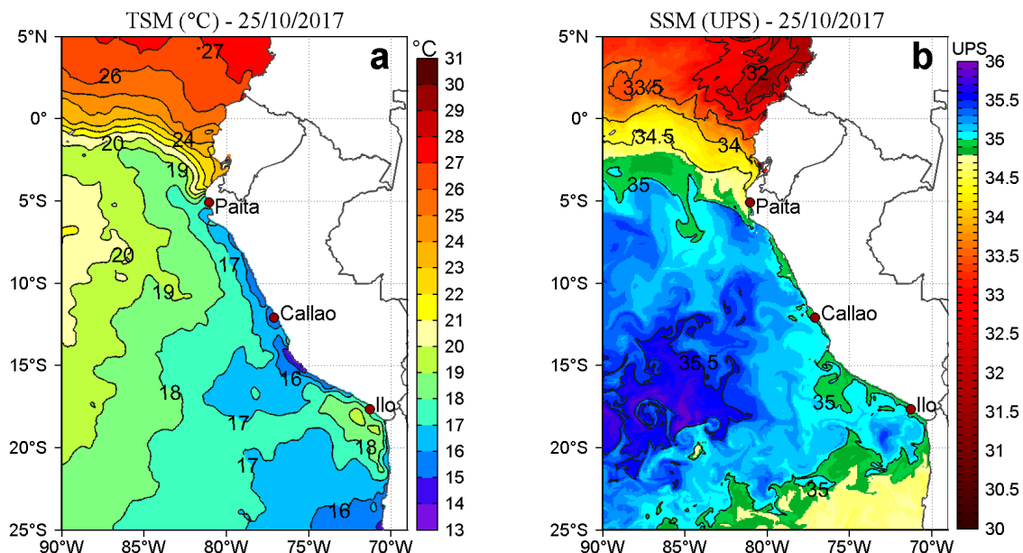
Figura 2. a) Temperatura superficial del mar ( ^{\circ}\text{C} ) y b) Salinidad superficial del mar (UPS) para el 25 de octubre. Datos: OSTIA-UKMO-L4-GLOB-v2.0 (UK Met Office, 2012; Donlon et al, 2012) disponible en https://podaac.jpl.nasa.gov/dataset/OSTIA-UKMO-L4-GLOB-v2.0 para (a) y Hybrid Coordinate Ocean Model (HYCOM; Halliwell et al., 1998; 2000; Bleck, 2001) para (b). Procesamiento: LHF/AFIOF/DGIOCC/IMARPE.
