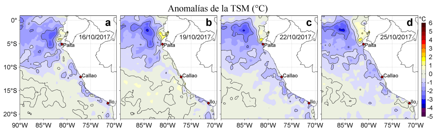
Figura 3. Anomalías de la Temperatura Superficial del Mar ( ^{\circ}\text{C} ) para los días: a) 16, b) 19, c) 22, y d) 25 de octubre de 2017. Las anomalías se calcularon respecto de la climatología para el periodo 2007-2016. Datos: OSTIA-UKMO-L4-GLOB-v2.0 (UK Met Office, 2012; Donlon et al, 2012). Procesamiento: LHF/AFIOF/DGIOCC/IMARPE.
