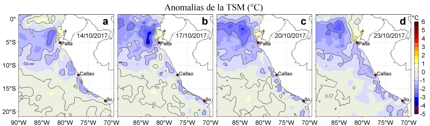
Figura 3. Anomalías de la Temperatura Superficial del Mar ( ^{\circ}\text{C} ) para los días: a) 14, b) 17, c) 20, y d) 23 de octubre de 2017. Las anomalías se calcularon respecto de la climatología para el periodo 2007-2016. Datos: OSTIA-UKMO-L4-GLOB-v2.0 (UK Met Office, 2012; Donlon et al, 2012). Procesamiento: LHF/AFIOF/DGIOCC/IMARPE.
