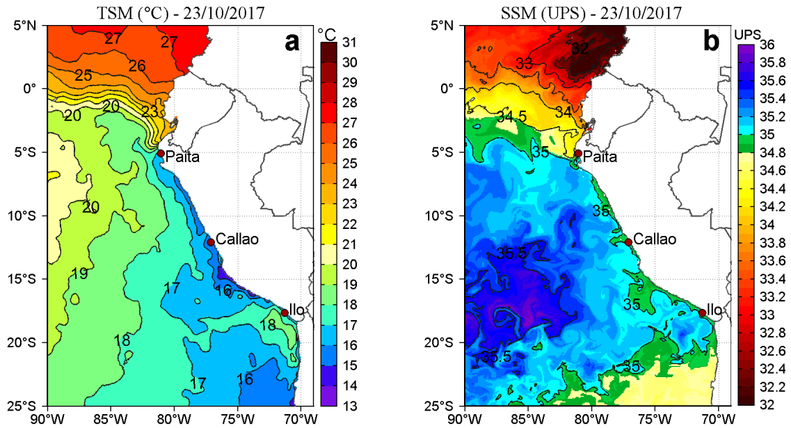
Figura 2. a) Temperatura superficial del mar ( ^{\circ}\text{C} ) y b) Salinidad superficial del mar (UPS) para el 23 de octubre. Datos: OSTIA-UKMO-L4-GLOB-v2.0 (UK Met Office, 2012; Donlon et al, 2012) disponible en https://podaac.jpl.nasa.gov/dataset/OSTIA-UKMO-L4-GLOB-v2.0 para (a) y Hybrid Coordinate Ocean Model (HYCOM; Halliwell et al., 1998; 2000; Bleck, 2001) para (b). Procesamiento: LHF/AFIOF/DGIOCC/IMARPE.
