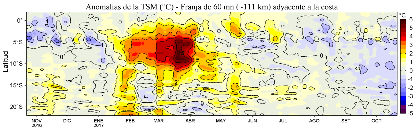
Figura 4. Variación promedio de las anomalías de la temperatura superficial del mar (°C) para una franja de 60 mn (~111 km) adyacente al litoral peruano para los últimos doce meses al 21 de octubre de 2017. Se distingue el calentamiento ocurrido de mediados de enero a fines de mayo de 2017 asociado con la presencia de El Niño Costero, evento que tuvo mayor impacto en la TSM (+5°C) en la segunda quincena de marzo. Datos: OSTIA-UKMO-L4-GLOB-v2.0 (UK Met. Office, 2012; Donlon et al, 2012) disponible en https://podaac.jpl.nasa.gov/dataset/OSTIA-UKMO-L4-GLOB-v2.0 . Las anomalías se calcularon con respecto al periodo 2007-2016. Procesamiento: LHF/AFIOF/DGIOCC/IMARPE.
