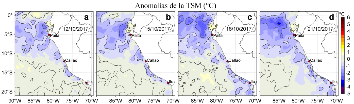
Figura 3. Anomalías de la Temperatura Superficial del Mar (°C) para los días: a) 12, b) 15, c) 18, y d) 21 de octubre de 2017. Las anomalías se calcularon respecto de la climatología para el periodo 2007-2016. Datos: OSTIA-UKMO-L4-GLOB-v2.0 (UK Met Office, 2012; Donlon et al, 2012). Procesamiento: LHF/AFIOF/DGIOCC/IMARPE.
