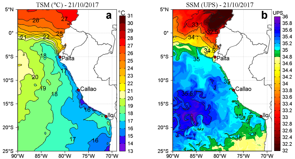
Figura 2. a) Temperatura superficial del mar (°C) y b) Salinidad superficial del mar (UPS) para el 21 de octubre. Datos: OSTIA-UKMO-L4-GLOB-v2.0 (UK Met Office, 2012; Donlon et al, 2012) disponible en https://podaac.jpl.nasa.gov/dataset/OSTIA-UKMO-L4-GLOB-v2.0 para (a) y Hybrid Coordinate Ocean Model (HYCOM; Halliwell et al., 1998; 2000; Bleck, 2001) para (b). Procesamiento: LHF/AFIOF/DGIOCC/IMARPE.
