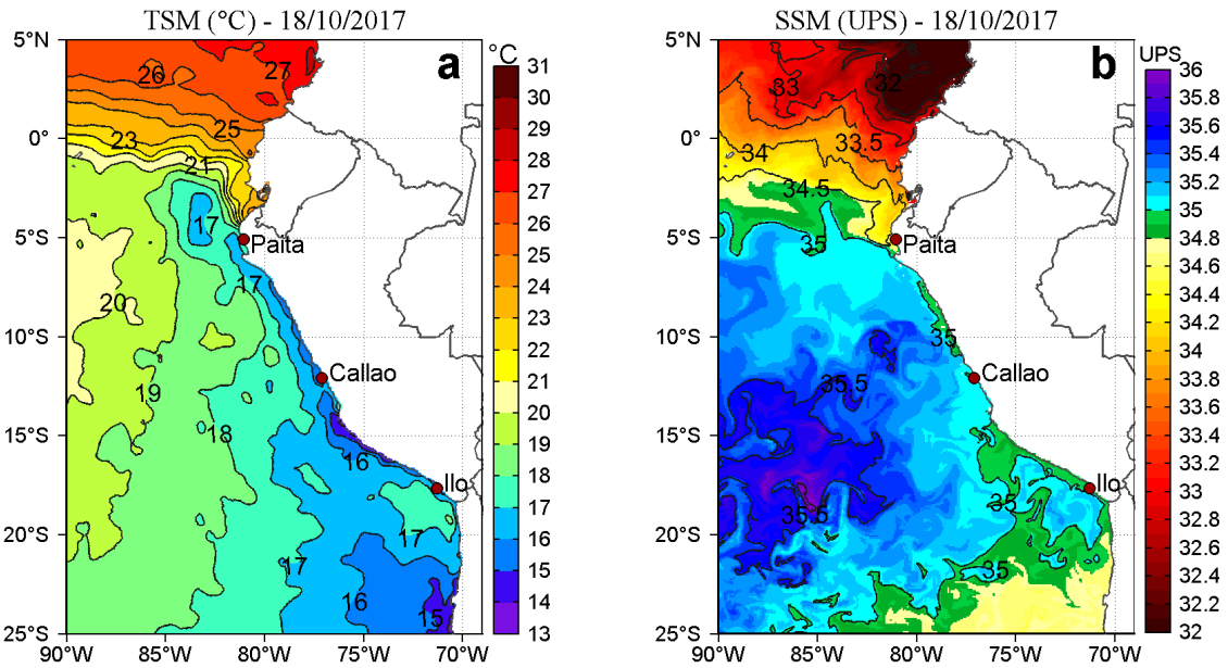
Figura 2. a) Temperatura superficial del mar ( ^{\circ}\text{C} ) y b) Salinidad superficial del mar (UPS) para el 18 de octubre. Datos: OSTIA-UKMO-L4-GLOB-v2.0 (UK Met Office, 2012; Donlon et al, 2012) disponible en https://podaac.jpl.nasa.gov/dataset/OSTIA-UKMO-L4-GLOB-v2.0 para (a) y Hybrid Coordinate Ocean Model (HYCOM; Halliwell et al., 1998; 2000; Bleck, 2001) para (b). Procesamiento: LHF/AFIOF/DGIOCC/IMARPE.
