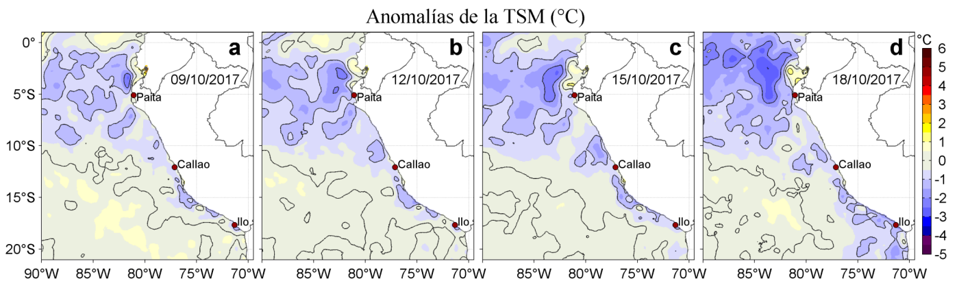
Figura 3. Anomalías de la Temperatura Superficial del Mar ( ^{\circ}\text{C} ) para los días: a) 09, b) 12, c) 15, y d) 18 de octubre de 2017. Las anomalías se calcularon respecto de la climatología para el periodo 2007-2016. Datos: OSTIA-UKMO-L4-GLOB-v2.0 (UK Met Office, 2012; Donlon et al, 2012). Procesamiento: LHF/AFIOF/DGIOCC/IMARPE.
