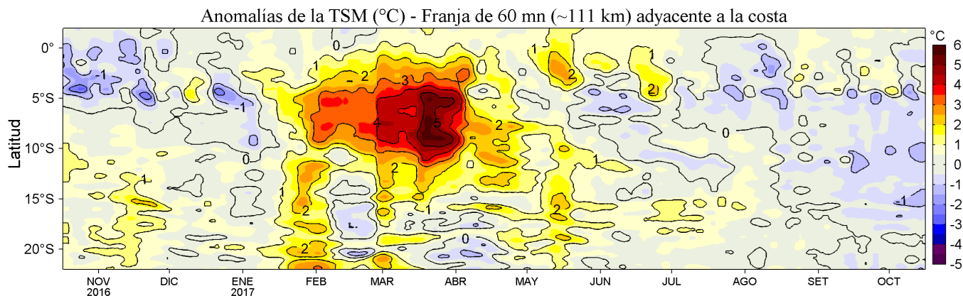
Figura 4. Variación promedio de las anomalías de la temperatura superficial del mar (°C) para una franja de 60 mn (~111 km) adyacente a la costa peruana para los últimos doce meses al 16 de octubre de 2017. Se distingue el calentamiento ocurrido de mediados de enero a fines de mayo de 2017 asociado con la presencia de El Niño Costero, evento que tuvo mayor impacto en la TSM (+5°C) en la segunda quincena de marzo. Datos: OSTIA-UKMO-L4-GLOB-v2.0 (UK Met. Office, 2012; Donlon et al, 2012) disponible en https://podaac.jpl.nasa.gov/dataset/OSTIA-UKMO-L4-GLOB-v2.0 ). Las anomalías se calcularon con respecto al periodo 2007-2016. Procesamiento: LHF/AFIOF/DGIOCC/IMARPE.
