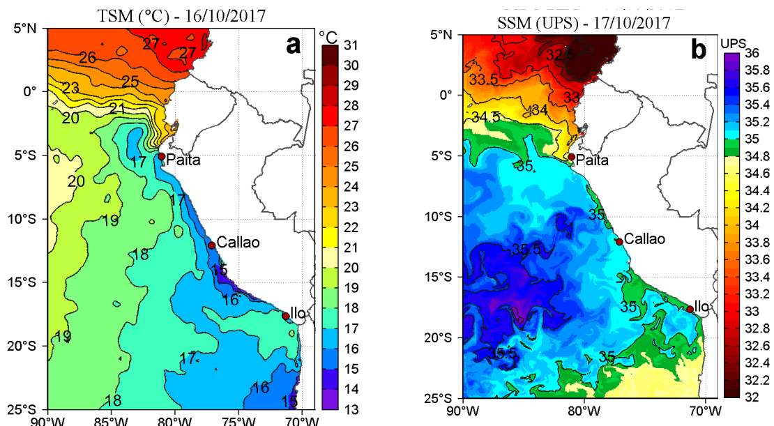
Figura 2. a) Temperatura superficial del mar (°C) y b) Salinidad superficial del mar (UPS) para el 16 y 17 de octubre respectivamente. Datos: OSTIA-UKMO-L4-GLOB-v2.0 (UK Met Office, 2012; Donlon et al, 2012) disponible en https://podaac.jpl.nasa.gov/dataset/OSTIA-UKMO-L4-GLOB-v2.0 para (a) y Hybrid Coordinate Ocean Model (HYCOM; Halliwell et al., 1998; 2000; Bleck, 2001) para (b). Procesamiento: LHF/AFIOF/DGIOCC/IMARPE.
