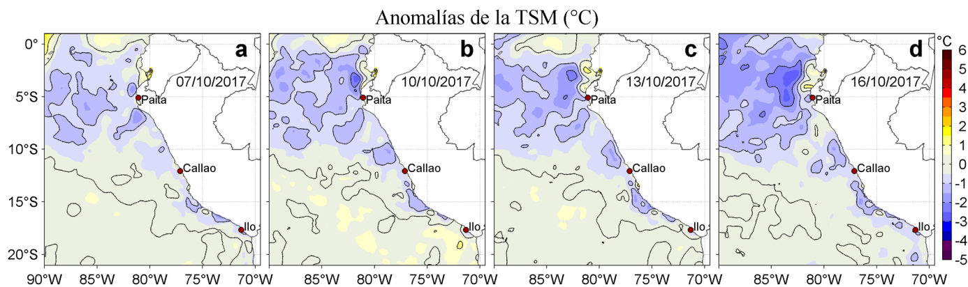
Figura 3. Anomalías de la Temperatura Superficial del Mar (°C) para los días: a) 07, b) 10, c) 13, y d) 16 de octubre de 2017. Las anomalías se calcularon respecto de la climatología para el periodo 2007-2016. Datos: OSTIA-UKMO-L4-GLOB-v2.0 (UK Met Office, 2012; Donlon et al, 2012). Procesamiento: LHF/AFIOF/DGIOCC/IMARPE.
