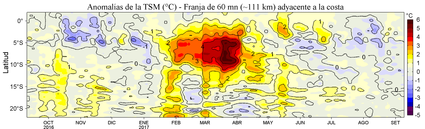
Figura 4. Variación promedio de las anomalías de la temperatura superficial del mar (°C) para una franja de 60 mn (~111 km) adyacente al litoral peruano para los últimos doce meses al 09 de setiembre de 2017. Se distingue el calentamiento ocurrido de mediados de enero a fines de mayo de 2017 asociado con la presencia de El Niño Costero, evento que tuvo mayor impacto en la TSM (+5°C) en la segunda quincena de marzo. Datos: OSTIA-UKMO-L4-GLOB-v2.0 (UK Met. Office, 2012; Donlon et al, 2012) disponible en https://podaac.jpl.nasa.gov/dataset/OSTIA-UKMO-L4-GLOB-v2.0 . Las anomalías se calcularon con respecto al periodo 2007-2016. Procesamiento: LHF/AFIOF/DGIOCC/IMARPE.
