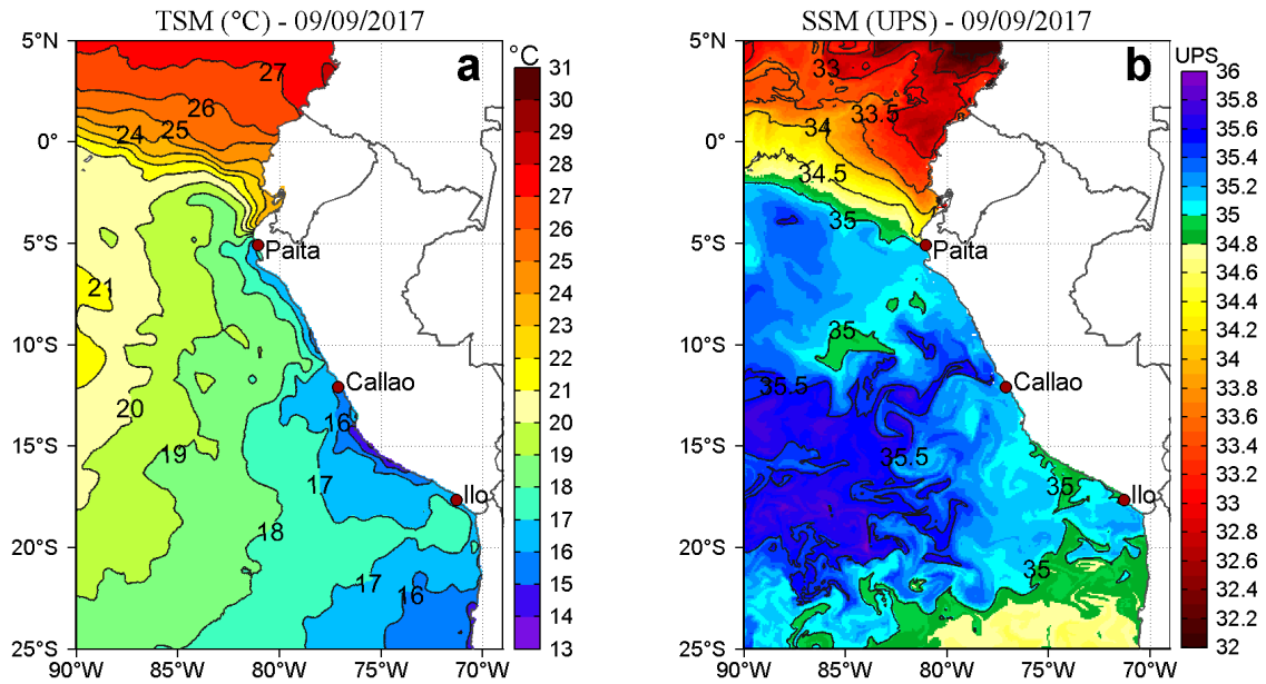
Figura 2. a) Temperatura superficial del mar (°C) y b) Salinidad superficial del mar (UPS) para el 09 de setiembre. Datos: OSTIA-UKMO-L4-GLOB-v2.0 (UK Met Office, 2012; Donlon et al, 2012) disponible en https://podaac.jpl.nasa.gov/dataset/OSTIA-UKMO-L4-GLOB-v2.0 para (a) y Hybrid Coordinate Ocean Model (HYCOM; Halliwell et al., 1998; 2000; Bleck, 2001) para (b). Procesamiento: LHF/AFIOF/DGIOCC/IMARPE.
