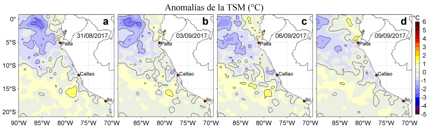
Figura 3. Anomalías de la Temperatura Superficial del Mar (°C) para los días: a) 31 de agosto, b) 03, c) 06 y d) 09 de setiembre de 2017. Las anomalías se calcularon respecto de la climatología para el periodo 2007-2016. Datos: OSTIA-UKMO-L4-GLOB-v2.0 (UK Met Office, 2012; Donlon et al, 2012). Procesamiento: LHF/AFIOF/DGIOCC/IMARPE.
