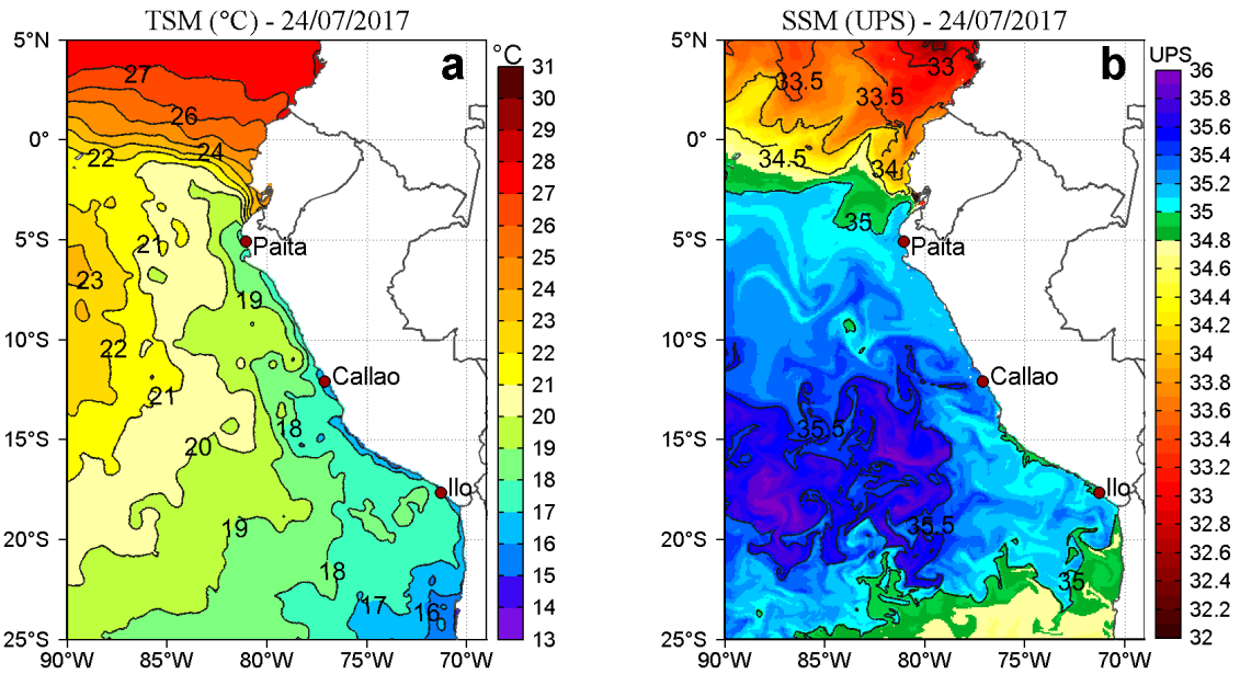
Figura 2. a) Temperatura superficial del mar (°C) y b) Salinidad superficial del mar (UPS) para el 24 de julio. Datos: OSTIA-UKMO-L4-GLOB-v2.0 (UK Met Office, 2012; Donlon et al, 2012) disponible en https://podaac.jpl.nasa.gov/dataset/OSTIA-UKMO-L4-GLOB-v2.0 para (a) y Hybrid Coordinate Ocean Model (HYCOM; Halliwell et al., 1998; 2000; Bleck, 2001) para (b). Procesamiento: LHF/AFIOF/DGIOCC/IMARPE.
