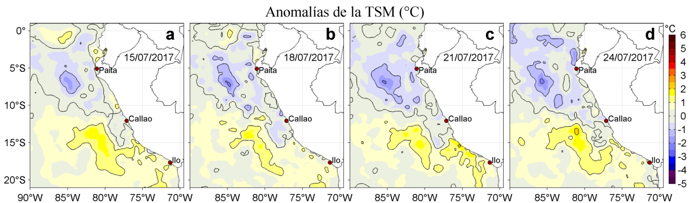
Figura 3. Anomalías de la Temperatura Superficial del Mar (°C) para los días: a) 15, b) 18, c) 21, y d) 24 de julio de 2017. Las anomalías se calcularon respecto de la climatología para el periodo 2007-2016. Datos: OSTIA-UKMO-L4-GLOB-v2.0 (UK Met Office, 2012; Donlon et al, 2012). Procesamiento: LHF/AFIOF/DGIOCC/IMARPE.
