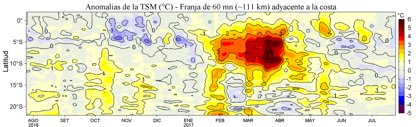
Figura 4. Variación promedio de las anomalías de la temperatura superficial del mar (°C) para una franja de 60 mn (~111 km) adyacente al litoral peruano para los últimos doce meses al 24 de julio de 2017. Se distingue el calentamiento ocurrido de mediados de enero a fines de mayo de 2017 asociado con la presencia de El Niño Costero, evento que tuvo mayor impacto en la TSM (+5°C) en la segunda quincena de marzo. Datos: OSTIA-UKMO-L4-GLOB-v2.0 (UK Met. Office, 2012; Donlon et al, 2012) disponible en https://podaac.jpl.nasa.gov/dataset/OSTIA-UKMO-L4-GLOB-v2.0 . Las anomalías se calcularon con respecto al periodo 2007-2016. Procesamiento: LHF/AFIOF/DGIOCC/IMARPE.
