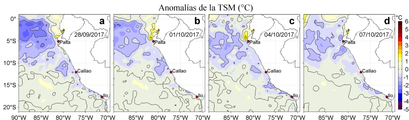
Figura 3. Anomalías de la Temperatura Superficial del Mar ( ^{\circ}\text{C} ) para los días: a) 28 de setiembre, b) 01, c) 04, y d) 07 de octubre de 2017. Las anomalías se calcularon respecto de la climatología para el periodo 2007-2016. Datos: OSTIA-UKMO-L4-GLOB-v2.0 (UK Met Office, 2012; Donlon et al, 2012). Procesamiento: LHF/AFIOF/DGIOCC/IMARPE.
