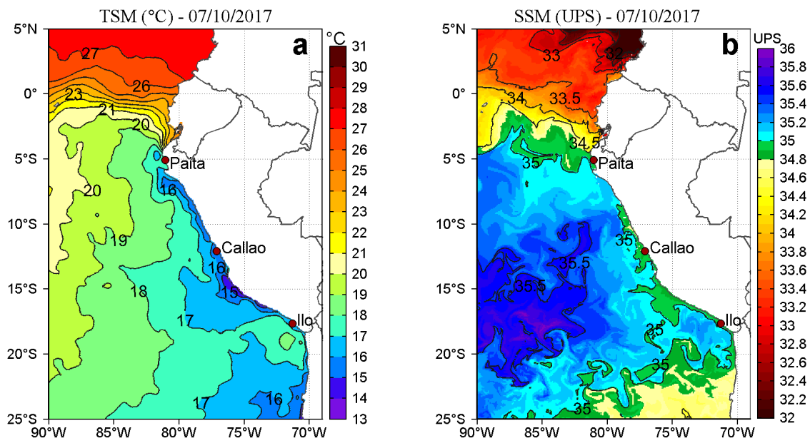
Figura 2. a) Temperatura superficial del mar ( ^{\circ}\text{C} ) y b) Salinidad superficial del mar (UPS) para el 07 de octubre. Datos: OSTIA-UKMO-L4-GLOB-v2.0 (UK Met Office, 2012; Donlon et al, 2012) disponible en https://podaac.jpl.nasa.gov/dataset/OSTIA-UKMO-L4-GLOB-v2.0 para (a) y Hybrid Coordinate Ocean Model (HYCOM; Halliwell et al., 1998; 2000; Bleck, 2001) para (b). Procesamiento: LHF/AFIOF/DGIOCC/IMARPE.
