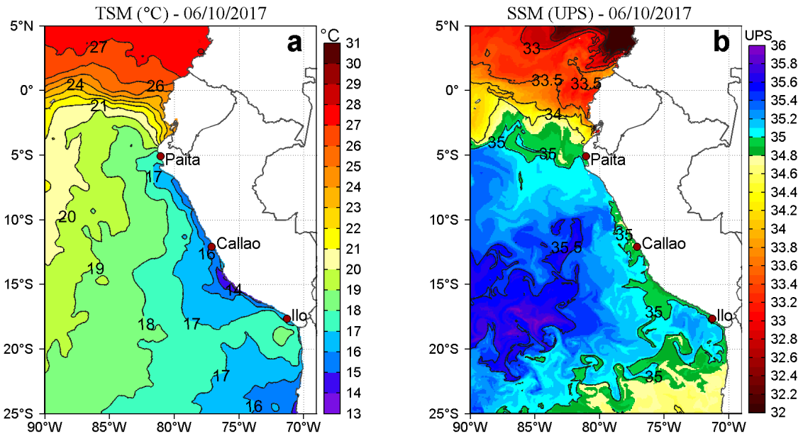
Figura 2. a) Temperatura superficial del mar ( ^{\circ}\text{C} ) y b) Salinidad superficial del mar (UPS) para el 06 de octubre. Datos: OSTIA-UKMO-L4-GLOB-v2.0 (UK Met Office, 2012; Donlon et al, 2012) disponible en https://podaac.jpl.nasa.gov/dataset/OSTIA-UKMO-L4-GLOB-v2.0 para (a) y Hybrid Coordinate Ocean Model (HYCOM; Halliwell et al., 1998; 2000; Bleck, 2001) para (b). Procesamiento: LHF/AFIOF/DGIOCC/IMARPE.
