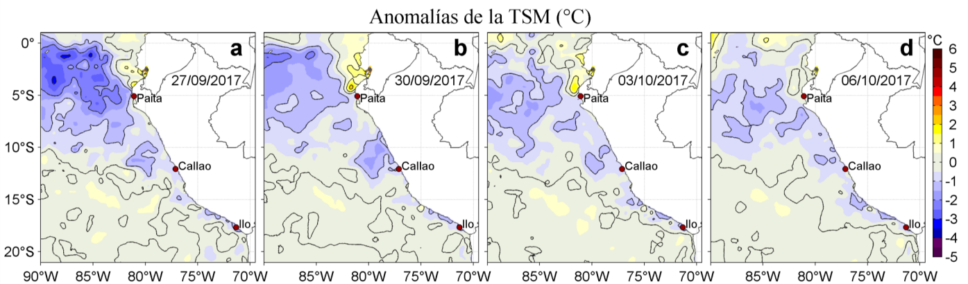
Figura 3. Anomalías de la Temperatura Superficial del Mar ( ^{\circ}\text{C} ) para los días: a) 27, b) 30, de setiembre, y c) 03, d) 06 de octubre de 2017. Las anomalías se calcularon respecto de la climatología para el periodo 2007-2016. Datos: OSTIA-UKMO-L4-GLOB-v2.0 (UK Met Office, 2012; Donlon et al, 2012). Procesamiento: LHF/AFIOF/DGIOCC/IMARPE.
