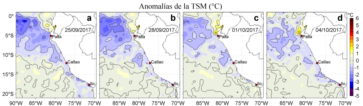
Figura 3. Anomalías de la Temperatura Superficial del Mar (°C) para los días: a) 25, b) 28, de setiembre, y c) 01, y d) 04 de octubre de 2017. Las anomalías se calcularon respecto de la climatología para el periodo 2007-2016. Datos: OSTIA-UKMO-L4-GLOB-v2.0 (UK Met Office, 2012; Donlon et al, 2012). Procesamiento: LHF/AFIOF/DGIOCC/IMARPE.
