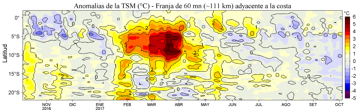
Figura 4. Variación promedio de las anomalías de la temperatura superficial del mar (°C) para una franja de 60 mn (~111 km) adyacente al litoral peruano para los últimos doce meses al 04 de octubre de 2017. Se distingue el calentamiento ocurrido de mediados de enero a fines de mayo de 2017 asociado con la presencia de El Niño Costero, evento que tuvo mayor impacto en la TSM (+5°C) en la segunda quincena de marzo. Datos: OSTIA-UKMO-L4-GLOB-v2.0 (UK Met. Office, 2012; Donlon et al, 2012) disponible en https://podaac.jpl.nasa.gov/dataset/OSTIA-UKMO-L4-GLOB-v2.0 ). Las anomalías se calcularon con respecto al periodo 2007-2016. Procesamiento: LHF/AFIOF/DGIOCC/IMARPE.
