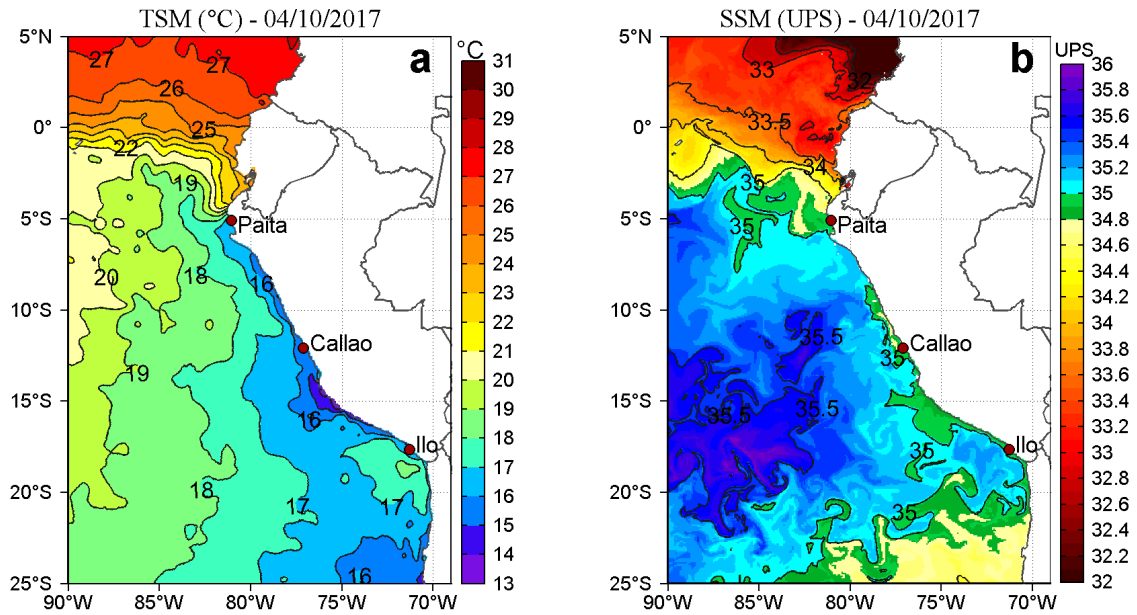
Figura 2. a) Temperatura superficial del mar (°C) y b) Salinidad superficial del mar (UPS) para el 04 de octubre. Datos: OSTIA-UKMO-L4-GLOB-v2.0 (UK Met Office, 2012; Donlon et al, 2012) disponible en https://podaac.jpl.nasa.gov/dataset/OSTIA-UKMO-L4-GLOB-v2.0 ) para (a) y Hybrid Coordinate Ocean Model (HYCOM; Halliwell et al., 1998; 2000; Bleck, 2001) para (b). Procesamiento: LHF/AFIOF/DGIOCC/IMARPE.
