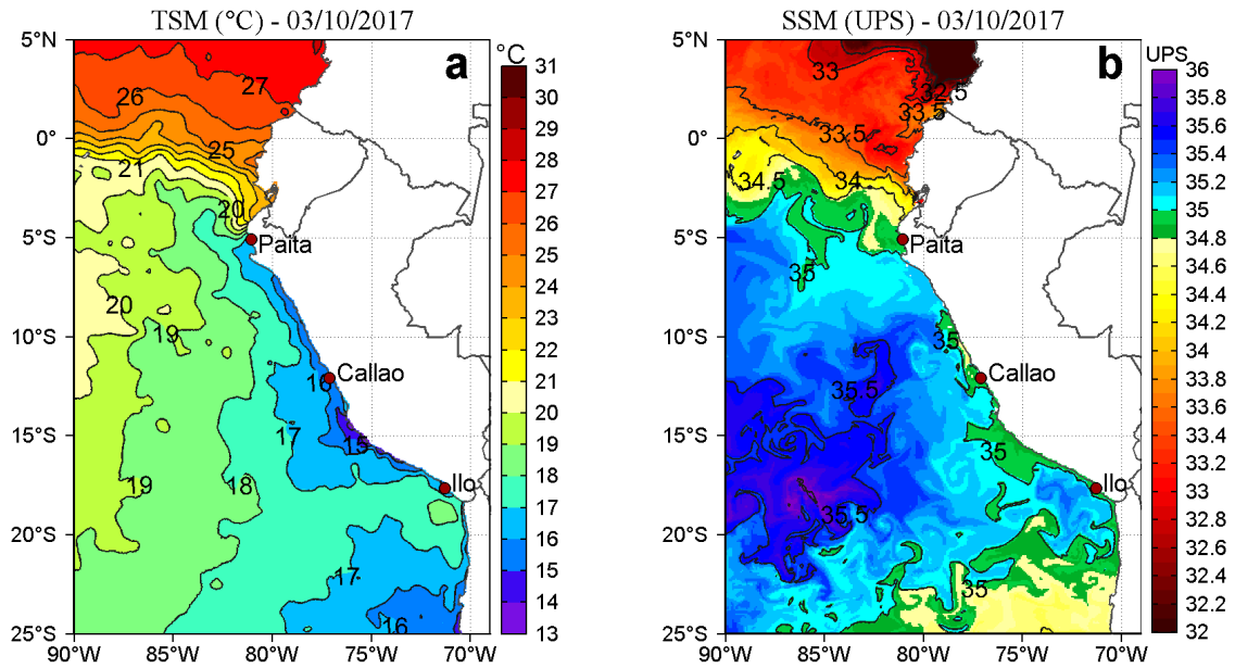
Figura 2. a) Temperatura superficial del mar (°C) y b) Salinidad superficial del mar (UPS) para el 03 de octubre. Datos: OSTIA-UKMO-L4-GLOB-v2.0 (UK Met Office, 2012; Donlon et al, 2012) disponible en https://podaac.jpl.nasa.gov/dataset/OSTIA-UKMO-L4-GLOB-v2.0 para (a) y Hybrid Coordinate Ocean Model (HYCOM; Halliwell et al., 1998; 2000; Bleck, 2001) para (b). Procesamiento: LHF/AFIOF/DGIOCC/IMARPE.
