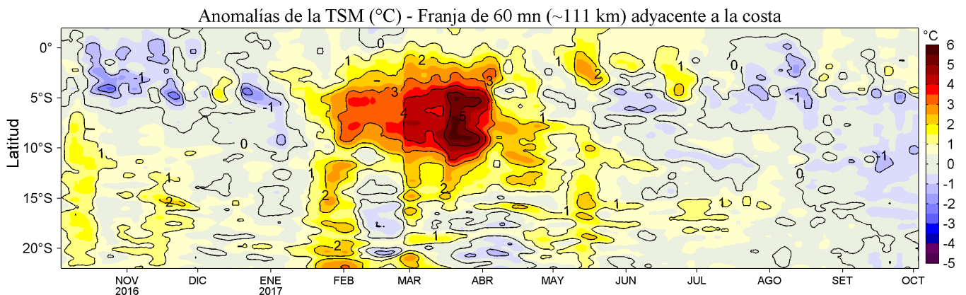
Figura 4. Variación promedio de las anomalías de la temperatura superficial del mar (°C) para una franja de 60 mn (~111 km) adyacente al litoral peruano para los últimos doce meses al 03 de octubre de 2017. Se distingue el calentamiento ocurrido de mediados de enero a fines de mayo de 2017 asociado con la presencia de El Niño Costero, evento que tuvo mayor impacto en la TSM (+5°C) en la segunda quincena de marzo. Datos: OSTIA-UKMO-L4-GLOB-v2.0 (UK Met. Office, 2012; Donlon et al, 2012) disponible en https://podaac.jpl.nasa.gov/dataset/OSTIA-UKMO-L4-GLOB-v2.0 ). Las anomalías se calcularon con respecto al periodo 2007-2016. Procesamiento: LHF/AFIOF/DGIOCC/IMARPE.
