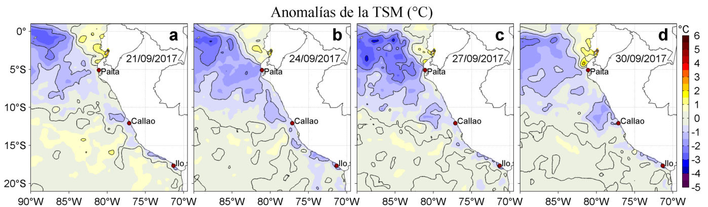
Figura 3. Anomalías de la Temperatura Superficial del Mar (°C) para los días: a) 21, b) 24, c) 27, y d) 30 de setiembre de 2017. Las anomalías se calcularon respecto de la climatología para el periodo 2007-2016. Datos: OSTIA-UKMO-L4-GLOB-v2.0 (UK Met Office, 2012; Donlon et al, 2012). Procesamiento: LHF/AFIOF/DGIOCC/IMARPE.
