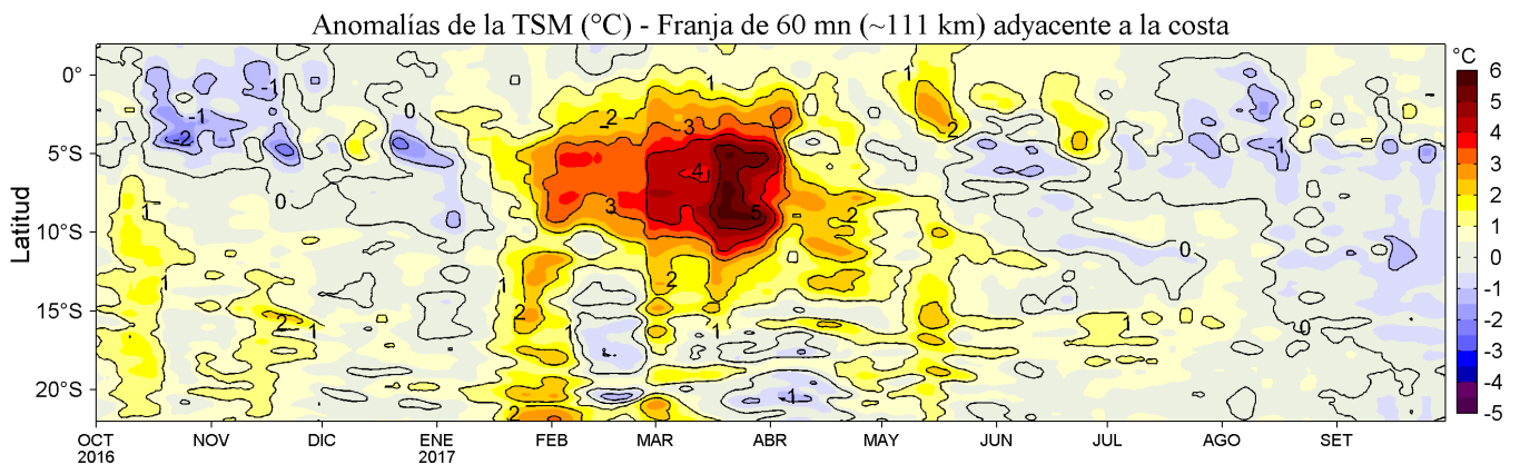
Figura 4. Variación promedio de las anomalías de la temperatura superficial del mar (°C) para una franja de 60 mn (~111 km) adyacente a la costa para los últimos doce meses al 30 de setiembre de 2017. Se distingue el calentamiento ocurrido de mediados de enero a fines de mayo de 2017 asociado con la presencia de El Niño Costero, evento que tuvo mayor impacto en la TSM (+5°C) en la segunda quincena de marzo. Datos: OSTIA-UKMO-L4-GLOB-v2.0 (UK Met. Office, 2012; Donlon et al, 2012) disponible en https://podaac.jpl.nasa.gov/dataset/OSTIA-UKMO-L4-GLOB-v2.0 . Las anomalías se calcularon con respecto al periodo 2007-2016. Procesamiento: LHF/AFIOF/DGIOCC/IMARPE.
