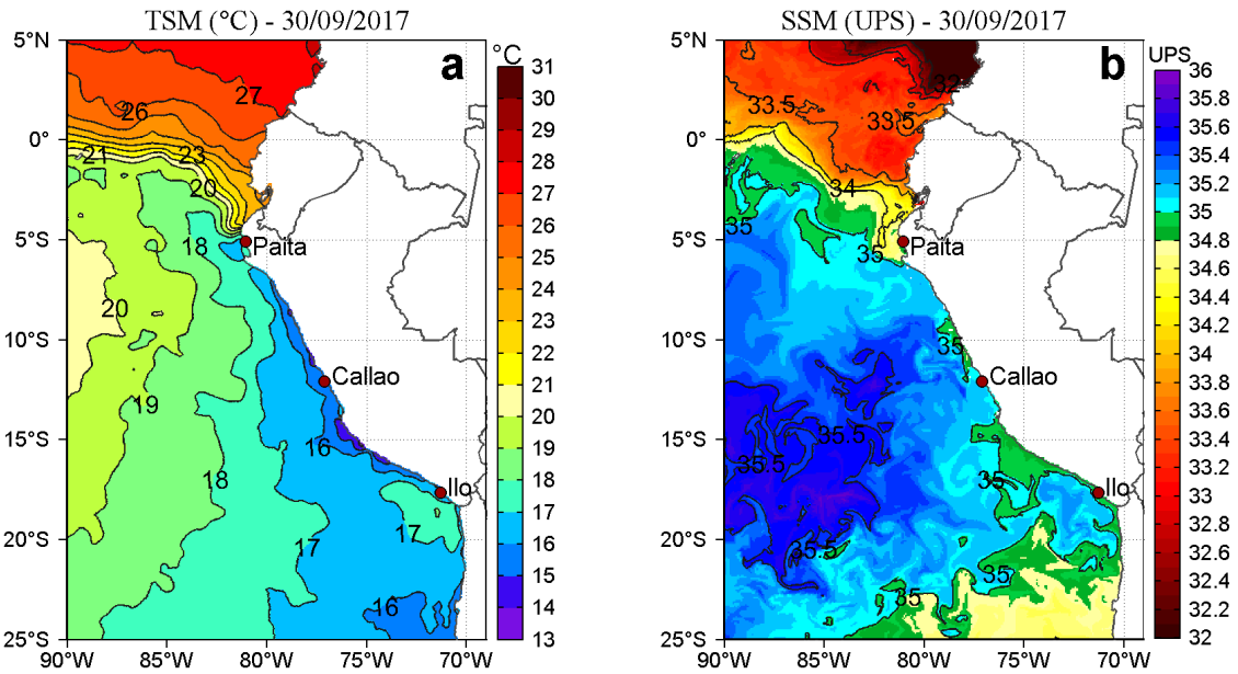
Figura 2. a) Temperatura superficial del mar (°C) y b) Salinidad superficial del mar (UPS) para el 30 de setiembre. Datos: OSTIA-UKMO-L4-GLOB-v2.0 (UK Met Office, 2012; Donlon et al, 2012) disponible en https://podaac.jpl.nasa.gov/dataset/OSTIA-UKMO-L4-GLOB-v2.0 para (a) y Hybrid Coordinate Ocean Model (HYCOM; Halliwell et al., 1998; 2000; Bleck, 2001) para (b). Procesamiento: LHF/AFIOF/DGIOCC/IMARPE.
