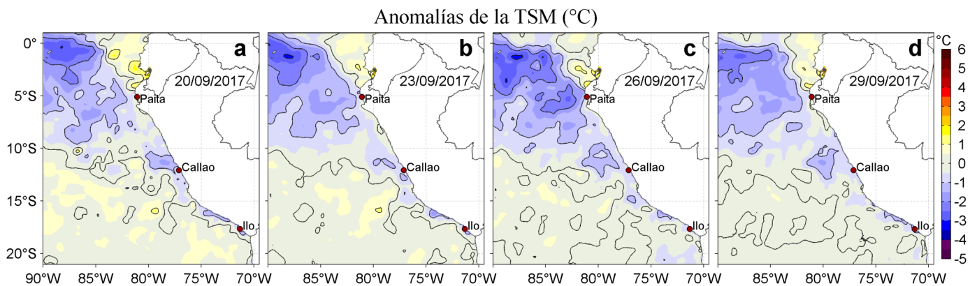
Figura 3. Anomalías de la Temperatura Superficial del Mar ( ^{\circ}\text{C} ) para los días: a) 20, b) 23, c) 26, y d) 29 de setiembre de 2017. Las anomalías se calcularon respecto de la climatología para el periodo 2007-2016. Datos: OSTIA-UKMO-L4-GLOB-v2.0 (UK Met Office, 2012; Donlon et al, 2012). Procesamiento: LHF/AFIOF/DGIOCC/IMARPE.
