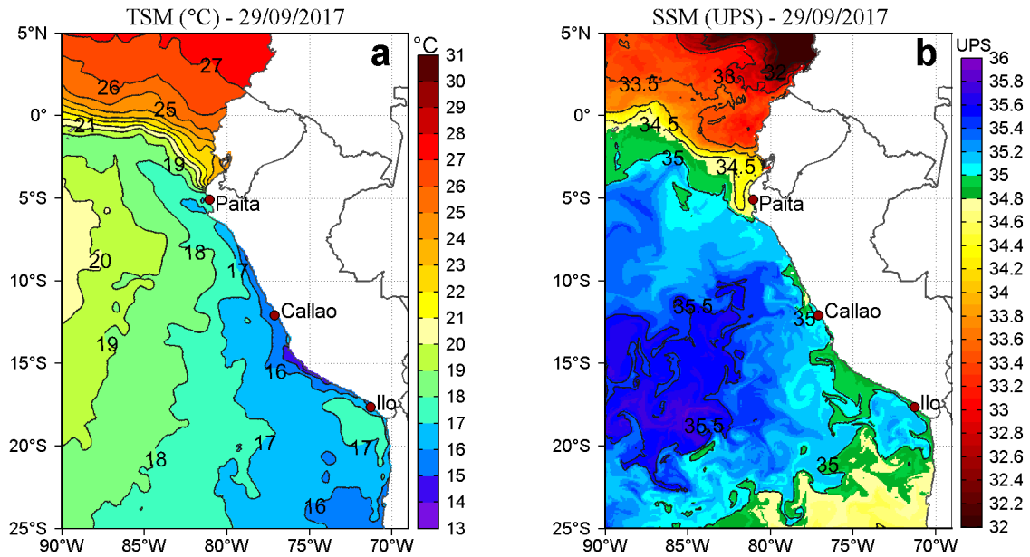
Figura 2. a) Temperatura superficial del mar ( ^{\circ}\text{C} ) y b) Salinidad superficial del mar (UPS) para el 29 de setiembre. Datos: OSTIA-UKMO-L4-GLOB-v2.0 (UK Met Office, 2012; Donlon et al, 2012) disponible en https://podaac.jpl.nasa.gov/dataset/OSTIA-UKMO-L4-GLOB-v2.0 para (a) y Hybrid Coordinate Ocean Model (HYCOM; Halliwell et al., 1998; 2000; Bleck, 2001) para (b). Procesamiento: LHF/AFIOF/DGIOCC/IMARPE.
