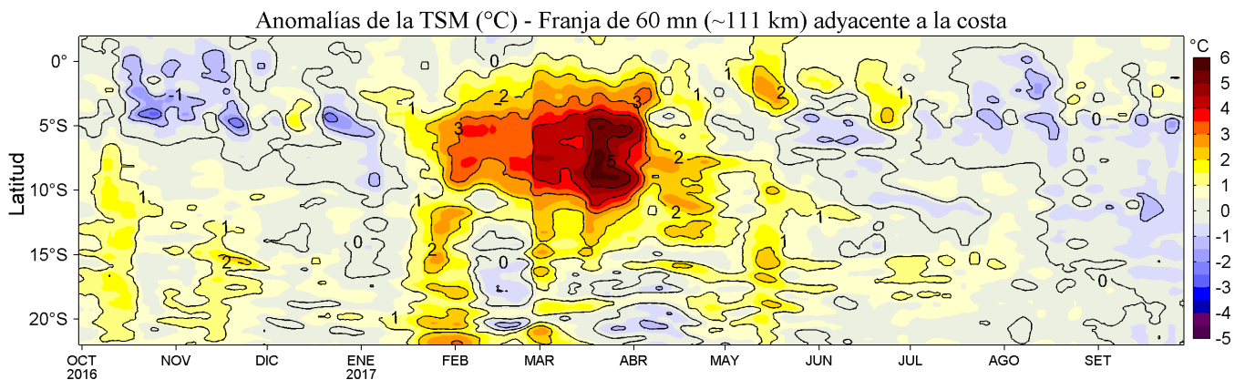
Figura 4. Variación promedio de las anomalías de la temperatura superficial del mar ( ^{\circ}\text{C} ) para una franja de 60 mn ( \sim 111 km) adyacente a la costa para los últimos doce meses al 29 de setiembre de 2017. Se distingue el calentamiento ocurrido de mediados de enero a fines de mayo de 2017 asociado con la presencia de El Niño Costero, evento que tuvo mayor impacto en la TSM ( +5^{\circ}\text{C} ) en la segunda quincena de marzo. Datos: OSTIA-UKMO-L4-GLOB-v2.0 (UK Met. Office, 2012; Donlon et al, 2012) disponible en https://podaac.jpl.nasa.gov/dataset/OSTIA-UKMO-L4-GLOB-v2.0 . Las anomalías se calcularon con respecto al periodo 2007-2016. Procesamiento: LHF/AFIOF/DGIOCC/IMARPE.
