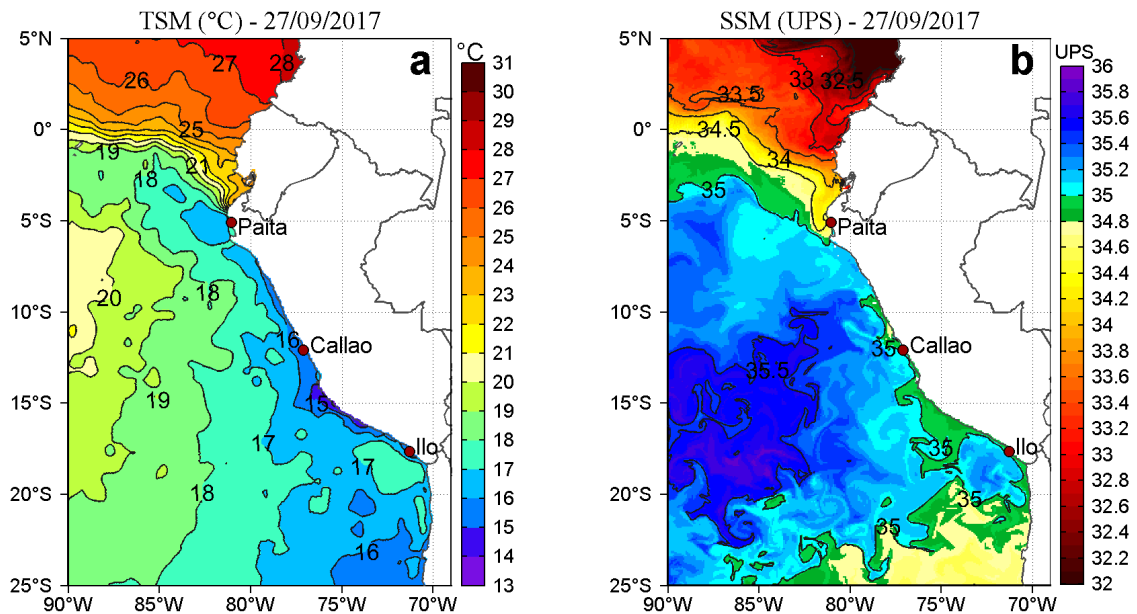
Figura 2. a) Temperatura superficial del mar ( ^{\circ}\text{C} ) y b) Salinidad superficial del mar (UPS) para el 27 de setiembre. Datos: OSTIA-UKMO-L4-GLOB-v2.0 (UK Met Office, 2012; Donlon et al, 2012) disponible en https://podaac.jpl.nasa.gov/dataset/OSTIA-UKMO-L4-GLOB-v2.0 para (a) y Hybrid Coordinate Ocean Model (HYCOM; Halliwell et al., 1998; 2000; Bleck, 2001) para (b). Procesamiento: LHFM/AFIOF/DGIOCC/IMARPE.
