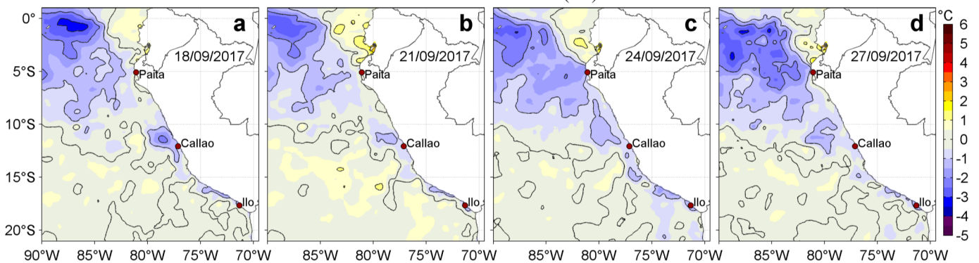
Figura 3. Anomalías de la Temperatura Superficial del Mar ( ^{\circ}\text{C} ) para los días: a) 18, b) 21, c) 24, y d) 27 de setiembre de 2017. Las anomalías se calcularon respecto de la climatología para el periodo 2007-2016. Datos: OSTIA-UKMO-L4-GLOB-v2.0 (UK Met Office, 2012; Donlon et al, 2012). Procesamiento: LHFM/AFIOF/DGIOCC/IMARPE.
