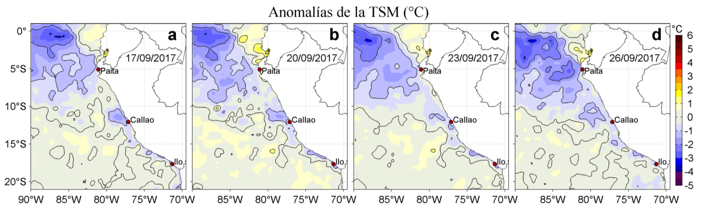
Figura 3. Anomalías de la Temperatura Superficial del Mar ( ^{\circ}\text{C} ) para los días: a) 17, b) 20, c) 23, y d) 26 de setiembre de 2017. Las anomalías se calcularon respecto de la climatología para el periodo 2007-2016. Datos: OSTIA-UKMO-L4-GLOB-v2.0 (UK Met Office, 2012; Donlon et al, 2012). Procesamiento: LHF/AFIOF/DGIOCC/IMARPE.
