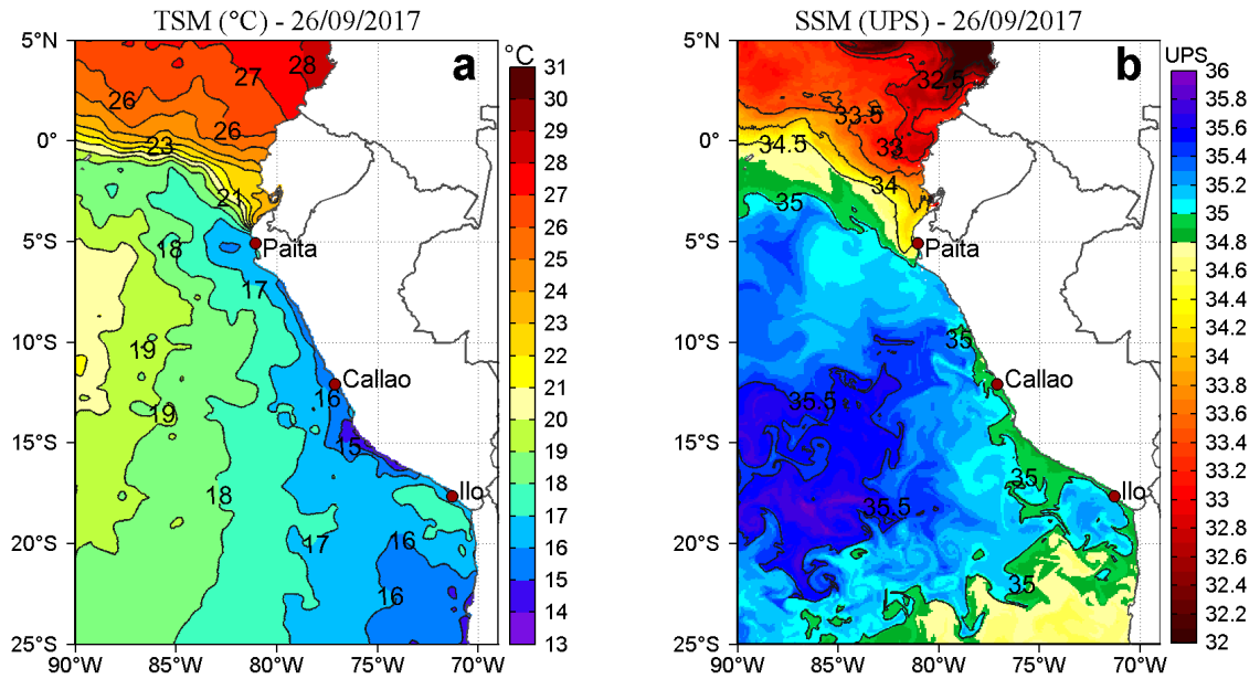
Figura 2. a) Temperatura superficial del mar ( ^{\circ}\text{C} ) y b) Salinidad superficial del mar (UPS) para el 26 de setiembre. Datos: OSTIA-UKMO-L4-GLOB-v2.0 (UK Met Office, 2012; Donlon et al, 2012) disponible en https://podaac.jpl.nasa.gov/dataset/OSTIA-UKMO-L4-GLOB-v2.0 para (a) y Hybrid Coordinate Ocean Model (HYCOM; Halliwell et al., 1998; 2000; Bleck, 2001) para (b). Procesamiento: LHF/AFIOF/DGIOCC/IMARPE.
