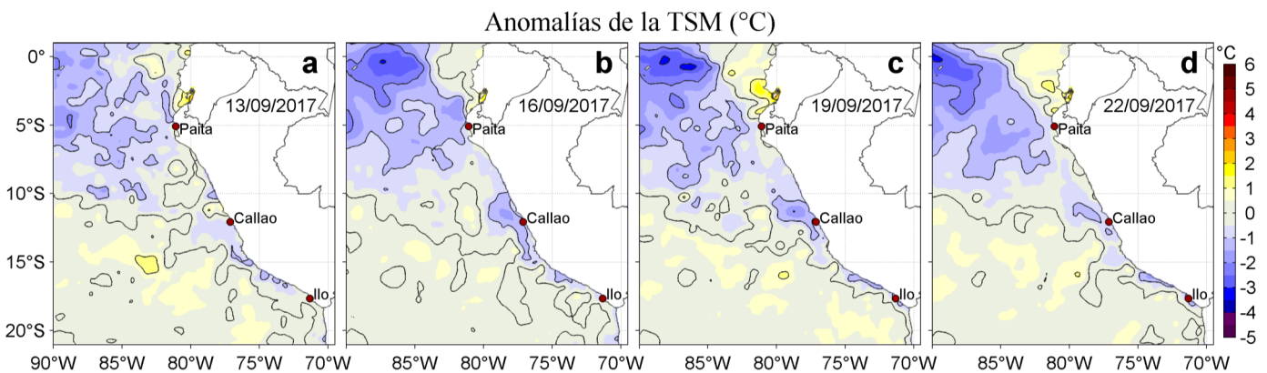
Figura 3. Anomalías de la Temperatura Superficial del Mar (°C) para los días: a) 13, b) 16, c) 19, y d) 22 de setiembre de 2017. Las anomalías se calcularon respecto de la climatología para el periodo 2007-2016. Datos: OSTIA-UKMO-L4-GLOB-v2.0 (UK Met Office, 2012; Donlon et al, 2012). Procesamiento: LHF/AFIOF/DGIOCC/IMARPE.
