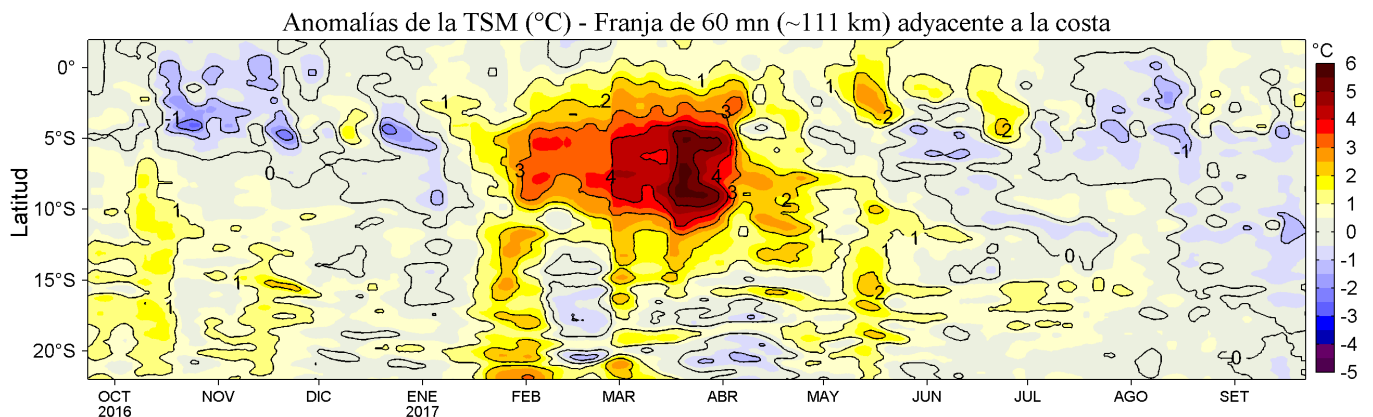
Figura 4. Variación promedio de las anomalías de la temperatura superficial del mar (°C) para una franja de 60 mn (~111 km) adyacente al litoral peruano para los últimos doce meses al 22 de setiembre de 2017. Se distingue el calentamiento ocurrido de mediados de enero a fines de mayo de 2017 asociado con la presencia de El Niño Costero, evento que tuvo mayor impacto en la TSM (+5°C) en la segunda quincena de marzo. Datos: OSTIA-UKMO-L4-GLOB-v2.0 (UK Met. Office, 2012; Donlon et al, 2012) disponible en https://podaac.jpl.nasa.gov/dataset/OSTIA-UKMO-L4-GLOB-v2.0 ). Las anomalías se calcularon con respecto al periodo 2007-2016. Procesamiento: LHF/AFIOF/DGIOCC/IMARPE.
