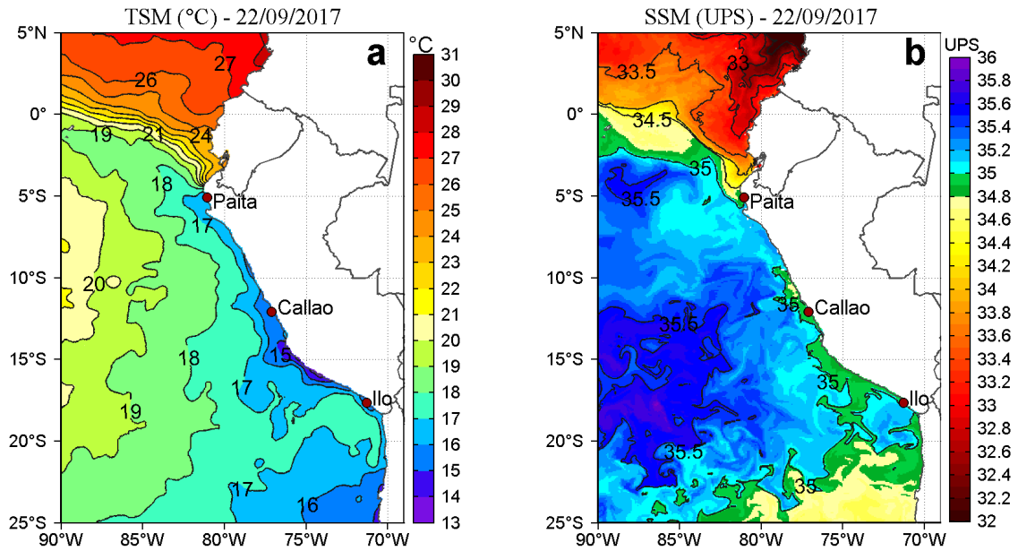
Figura 2. a) Temperatura superficial del mar (°C) y b) Salinidad superficial del mar (UPS) para el 22 de setiembre. Datos: OSTIA-UKMO-L4-GLOB-v2.0 (UK Met Office, 2012; Donlon et al, 2012) disponible en https://podaac.jpl.nasa.gov/dataset/OSTIA-UKMO-L4-GLOB-v2.0 para (a) y Hybrid Coordinate Ocean Model (HYCOM; Halliwell et al., 1998; 2000; Bleck, 2001) para (b). Procesamiento: LHF/AFIOF/DGIOCC/IMARPE.
