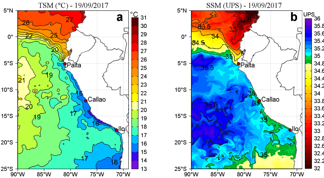
Figura 2. a) Temperatura superficial del mar (°C) y b) Salinidad superficial del mar (UPS) para el 19 de setiembre. Datos: OSTIA-UKMO-L4-GLOB-v2.0 (UK Met Office, 2012; Donlon et al, 2012) disponible en https://podaac.jpl.nasa.gov/dataset/OSTIA-UKMO-L4-GLOB-v2.0 para (a) y Hybrid Coordinate Ocean Model (HYCOM; Halliwell et al., 1998; 2000; Bleck, 2001) para (b). Procesamiento: LHF/AFIOF/DGIOCC/IMARPE.
