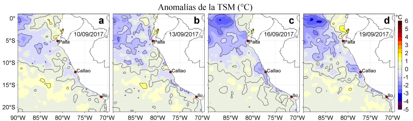
Figura 3. Anomalías de la Temperatura Superficial del Mar (°C) para los días: a) 10, b) 13, c) 16, y d) 19 de setiembre de 2017. Las anomalías se calcularon respecto de la climatología para el periodo 2007-2016. Datos: OSTIA-UKMO-L4-GLOB-v2.0 (UK Met Office, 2012; Donlon et al, 2012). Procesamiento: LHF/AFIOF/DGIOCC/IMARPE.
