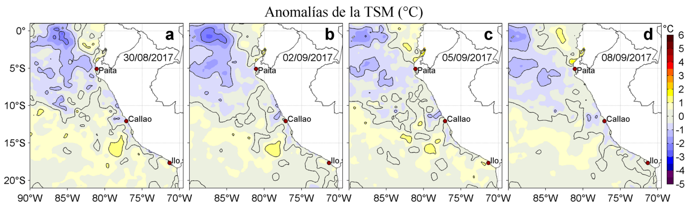
Figura 3. Anomalías de la Temperatura Superficial del Mar ( ^{\circ}\text{C} ) para los días: a) 30 de agosto, b) 02, c) 05 y d) 08 de setiembre de 2017. Las anomalías se calcularon respecto de la climatología para el periodo 2007-2016. Datos: OSTIA-UKMO-L4-GLOB-v2.0 (UK Met Office, 2012; Donlon et al, 2012). Procesamiento: LHF/AFIOF/DGIOCC/IMARPE.
