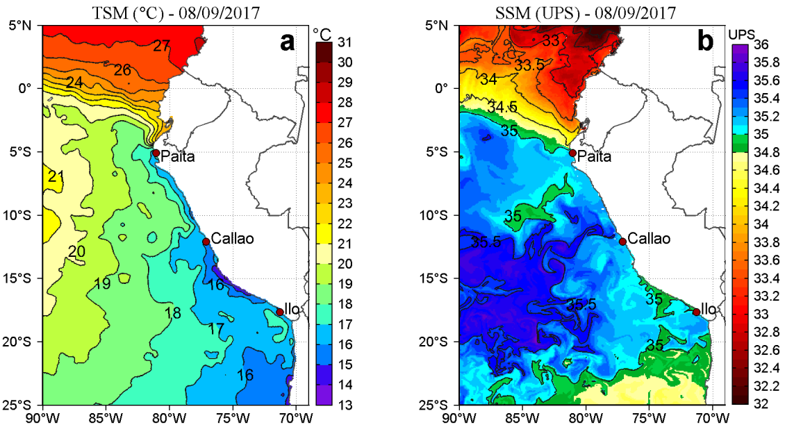
Figura 2. a) Temperatura superficial del mar ( ^{\circ}\text{C} ) y b) Salinidad superficial del mar (UPS) para el 08 de setiembre. Datos: OSTIA-UKMO-L4-GLOB-v2.0 (UK Met Office, 2012; Donlon et al, 2012) disponible en https://podaac.jpl.nasa.gov/dataset/OSTIA-UKMO-L4-GLOB-v2.0 para (a) y Hybrid Coordinate Ocean Model (HYCOM; Halliwell et al., 1998; 2000; Bleck, 2001) para (b). Procesamiento: LHF/AFIOF/DGIOCC/IMARPE.
