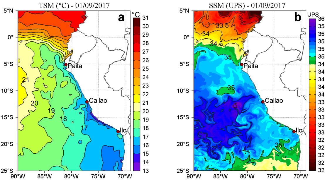
Figura 2. a) Temperatura superficial del mar ( ^{\circ}\text{C} ) y b) Salinidad superficial del mar (UPS) para el 01 de setiembre. Datos: OSTIA-UKMO-L4-GLOB-v2.0 (UK Met Office, 2012; Donlon et al, 2012) disponible en https://podaac.jpl.nasa.gov/dataset/OSTIA-UKMO-L4-GLOB-v2.0 para (a) y Hybrid Coordinate Ocean Model (HYCOM; Halliwell et al., 1998; 2000; Bleck, 2001) para (b). Procesamiento: LHF/AFIOF/DGIOCC/IMARPE.
