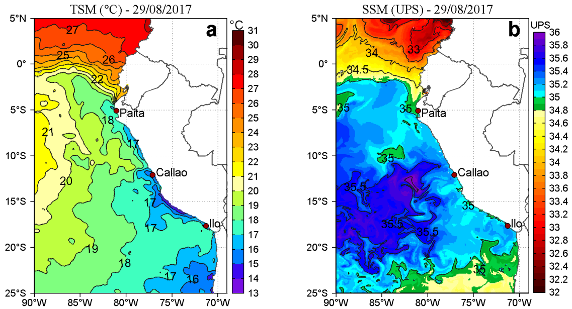
Figura 2. a) Temperatura superficial del mar (°C) y b) Salinidad superficial del mar (UPS) para el 29 de agosto respectivamente. Datos: OSTIA-UKMO-L4-GLOB-v2.0 (UK Met Office, 2012; Donlon et al, 2012) disponible en https://podaac.jpl.nasa.gov/dataset/OSTIA-UKMO-L4-GLOB-v2.0 para (a) y Hybrid Coordinate Ocean Model (HYCOM; Halliwell et al., 1998; 2000; Bleck, 2001) para (b). Procesamiento: LHF/AFIOF/DGIOCC/IMARPE.
