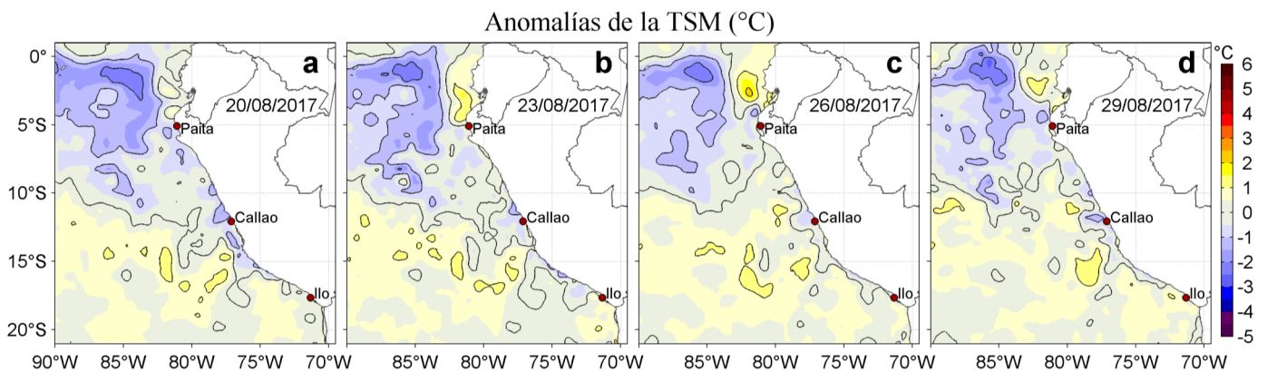
Figura 3. Anomalías de la Temperatura Superficial del Mar (°C) para los días: a) 20, b) 23, c) 26, y d) 29 de agosto de 2017. Las anomalías se calcularon respecto de la climatología para el periodo 2007-2016. Datos: OSTIA-UKMO-L4-GLOB-v2.0 (UK Met Office, 2012; Donlon et al, 2012). Procesamiento: LHF/AFIOF/DGIOCC/IMARPE.
