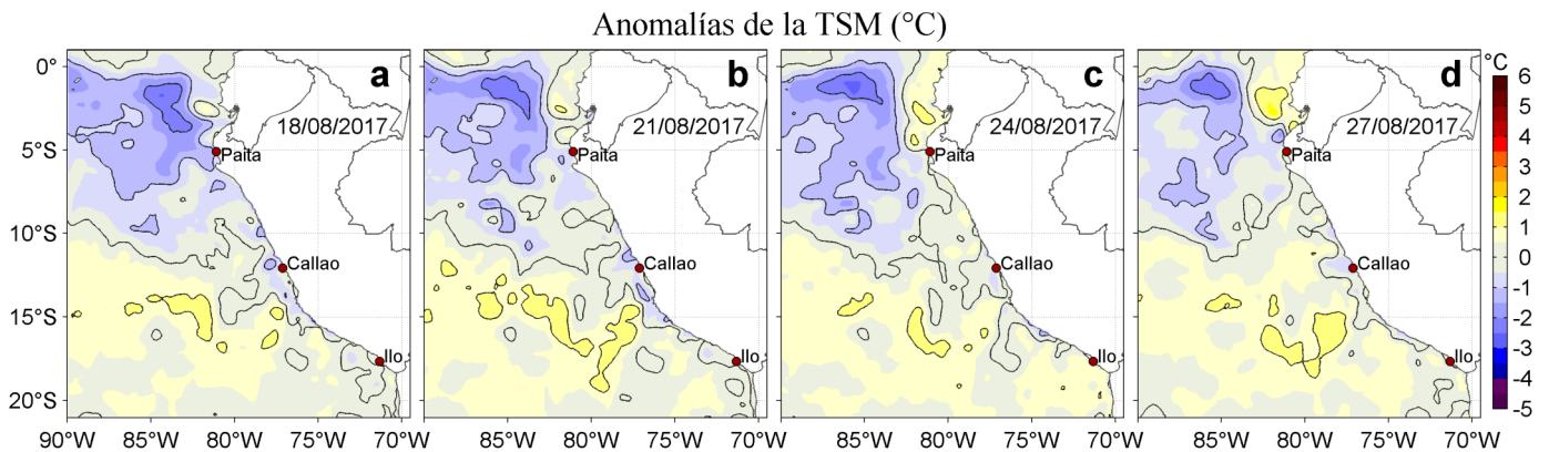
Figura 3. Anomalías de la Temperatura Superficial del Mar ( ^{\circ}\text{C} ) para los días: a) 18, b) 21, c) 24, y d) 27 de agosto de 2017. Las anomalías se calcularon respecto de la climatología para el periodo 2007-2016. Datos: OSTIA-UKMO-L4-GLOB-v2.0 (UK Met Office, 2012; Donlon et al, 2012). Procesamiento: LHF/AFIOF/DGIOCC/IMARPE.
