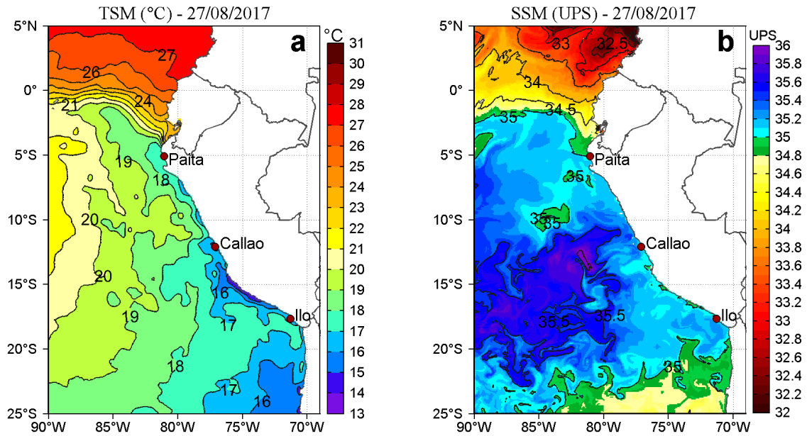
Figura 2. a) Temperatura superficial del mar ( ^{\circ}\text{C} ) y b) Salinidad superficial del mar (UPS) para el 27 de agosto respectivamente. Datos: OSTIA-UKMO-L4-GLOB-v2.0 (UK Met Office, 2012; Donlon et al, 2012) disponible en https://podaac.jpl.nasa.gov/dataset/OSTIA-UKMO-L4-GLOB-v2.0 para (a) y Hybrid Coordinate Ocean Model (HYCOM; Halliwell et al., 1998; 2000; Bleck, 2001) para (b). Procesamiento: LHF/AFIOF/DGIOCC/IMARPE.
