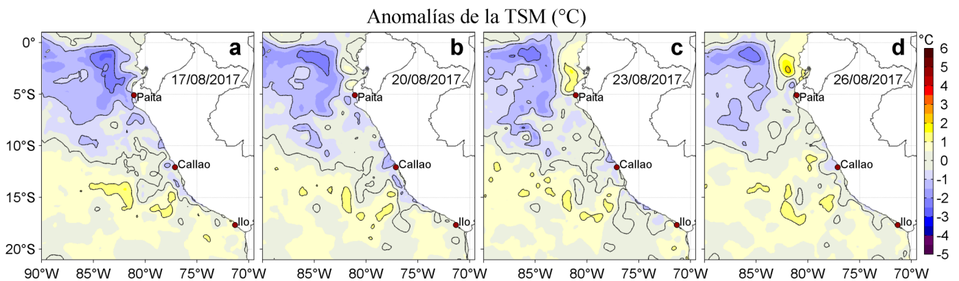
Figura 3. Anomalías de la Temperatura Superficial del Mar (°C) para los días: a) 17, b) 20, c) 23, y d) 26 de agosto de 2017. Las anomalías se calcularon respecto de la climatología para el periodo 2007-2016. Datos: OSTIA-UKMO-L4-GLOB-v2.0 (UK Met Office, 2012; Donlon et al, 2012). Procesamiento: LHF/AFIOF/DGIOCC/IMARPE.
