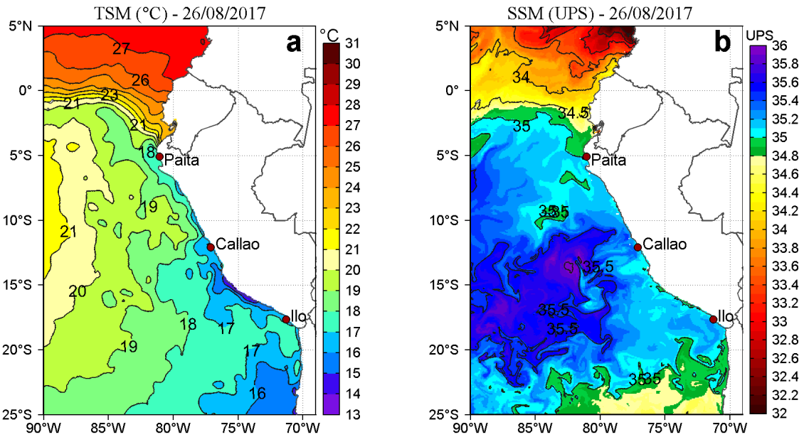
Figura 2. a) Temperatura superficial del mar (°C) y b) Salinidad superficial del mar (UPS) para el 26 de agosto respectivamente. Datos: OSTIA-UKMO-L4-GLOB-v2.0 (UK Met Office, 2012; Donlon et al, 2012) disponible en https://podaac.jpl.nasa.gov/dataset/OSTIA-UKMO-L4-GLOB-v2.0 para (a) y Hybrid Coordinate Ocean Model (HYCOM; Halliwell et al., 1998; 2000; Bleck, 2001) para (b). Procesamiento: LHF/AFIOF/DGIOCC/IMARPE.
