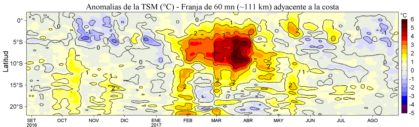
Figura 4. Variación promedio de las anomalías de la temperatura superficial del mar (°C) para una franja de 60 mn (~111 km) adyacente al litoral peruano para los últimos doce meses al 26 de agosto de 2017. Se distingue el calentamiento ocurrido de mediados de enero a fines de mayo de 2017 asociado con la presencia de El Niño Costero, evento que tuvo mayor impacto en la TSM (+5°C) en la segunda quincena de marzo. Datos: OSTIA-UKMO-L4-GLOB-v2.0 (UK Met Office, 2012; Donlon et al, 2012) disponible en https://podaac.jpl.nasa.gov/dataset/OSTIA-UKMO-L4-GLOB-v2.0 . Las anomalías se calcularon con respecto al periodo 2007-2016. Procesamiento: LHF/AFIOF/DGIOCC/IMARPE.
