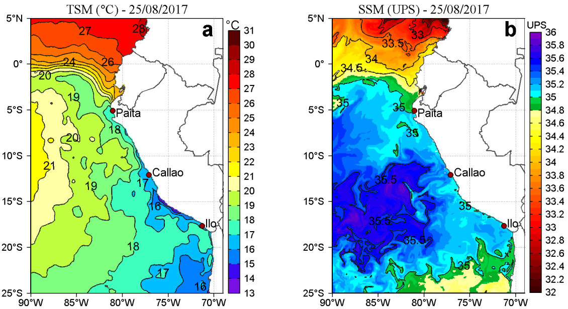
Figura 2. a) Temperatura superficial del mar ( ^{\circ}\text{C} ) y b) Salinidad superficial del mar (UPS) para el 25 de agosto respectivamente. Datos: OSTIA-UKMO-L4-GLOB-v2.0 (UK Met Office, 2012; Donlon et al, 2012) disponible en https://podaac.jpl.nasa.gov/dataset/OSTIA-UKMO-L4-GLOB-v2.0 para (a) y Hybrid Coordinate Ocean Model (HYCOM; Halliwell et al., 1998; 2000; Bleck, 2001) para (b). Procesamiento: LHF/AFIOF/DGIOCC/IMARPE.
