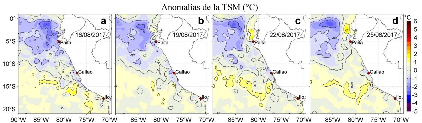
Figura 3. Anomalías de la Temperatura Superficial del Mar ( ^{\circ}\text{C} ) para los días: a) 16, b) 19, c) 22, y d) 25 de agosto de 2017. Las anomalías se calcularon respecto de la climatología para el periodo 2007-2016. Datos: OSTIA-UKMO-L4-GLOB-v2.0 (UK Met Office, 2012; Donlon et al, 2012). Procesamiento: LHF/AFIOF/DGIOCC/IMARPE.
