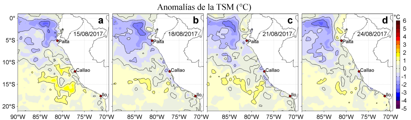
Figura 3. Anomalías de la Temperatura Superficial del Mar ( ^{\circ}\text{C} ) para los días: a) 15, b) 18, c) 21, y d) 24 de agosto de 2017. Las anomalías se calcularon respecto de la climatología para el periodo 2007-2016. Datos: OSTIA-UKMO-L4-GLOB-v2.0 (UK Met Office, 2012; Donlon et al, 2012). Procesamiento: LHF/AFIOF/DGIOCC/IMARPE.
