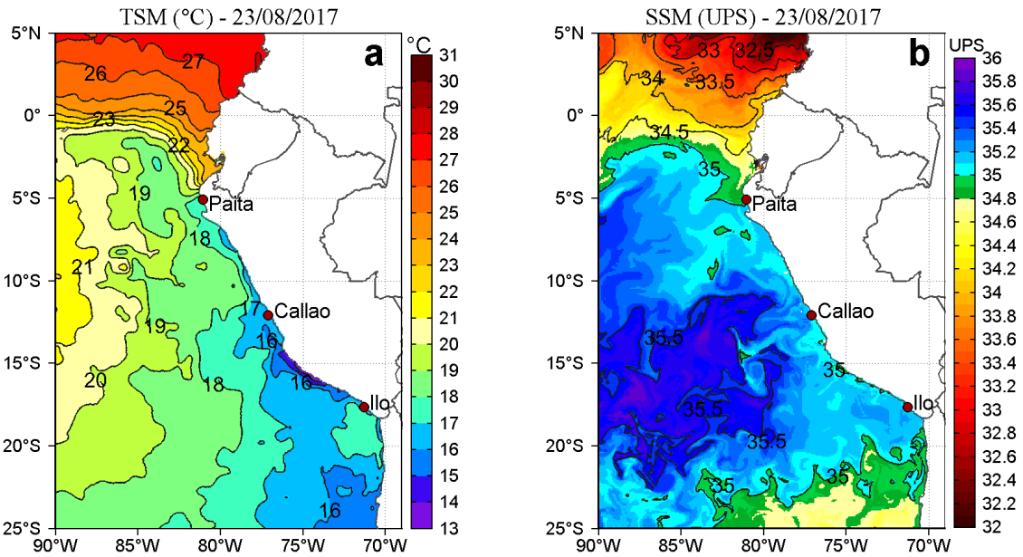
Figura 2. a) Temperatura superficial del mar ( ^{\circ}\text{C} ) y b) Salinidad superficial del mar (UPS) para el 23 de agosto respectivamente. Datos: OSTIA-UKMO-L4-GLOB-v2.0 (UK Met Office, 2012; Donlon et al, 2012) disponible en https://podaac.jpl.nasa.gov/dataset/OSTIA-UKMO-L4-GLOB-v2.0 para (a) y Hybrid Coordinate Ocean Model (HYCOM; Halliwell et al., 1998; 2000; Bleck, 2001) para (b). Procesamiento: LHF/AFIOF/DGIOCC/IMARPE.
