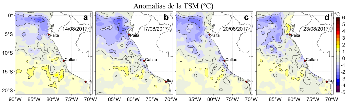
Figura 3. Anomalías de la Temperatura Superficial del Mar ( ^{\circ}\text{C} ) para los días: a) 14, b) 17, c) 20, y d) 23 de agosto de 2017. Las anomalías se calcularon respecto de la climatología para el periodo 2007-2016. Datos: OSTIA-UKMO-L4-GLOB-v2.0 (UK Met Office, 2012; Donlon et al, 2012). Procesamiento: LHF/AFIOF/DGIOCC/IMARPE.
