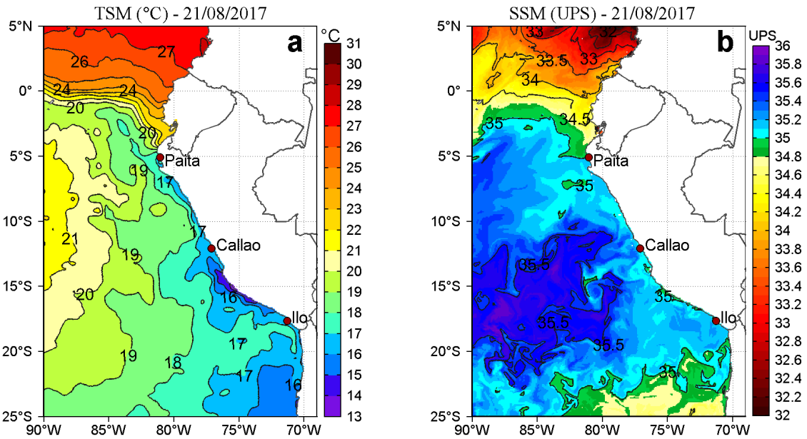
Figura 2. a) Temperatura superficial del mar ( ^{\circ}\text{C} ) y b) Salinidad superficial del mar (UPS) para el 21 de agosto respectivamente. Datos: OSTIA-UKMO-L4-GLOB-v2.0 (UK Met Office, 2012; Donlon et al, 2012) disponible en https://podaac.jpl.nasa.gov/dataset/OSTIA-UKMO-L4-GLOB-v2.0 para (a) y Hybrid Coordinate Ocean Model (HYCOM; Halliwell et al., 1998; 2000; Bleck, 2001) para (b). Procesamiento: LHF/AFIOF/DGIOCC/IMARPE.
