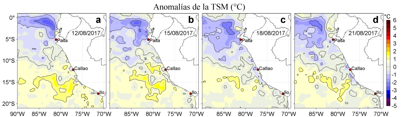
Figura 3. Anomalías de la Temperatura Superficial del Mar ( ^{\circ}\text{C} ) para los días: a) 12, b) 15, c) 18, y d) 21 de agosto de 2017. Las anomalías se calcularon respecto de la climatología para el periodo 2007-2016. Datos: OSTIA-UKMO-L4-GLOB-v2.0 (UK Met Office, 2012; Donlon et al, 2012). Procesamiento: LHF/AFIOF/DGIOCC/IMARPE.
