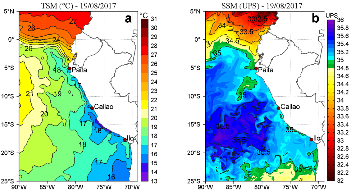
Figura 2. a) Temperatura superficial del mar ( ^{\circ}\text{C} ) y b) Salinidad superficial del mar (UPS) para el 19 de agosto respectivamente. Datos: OSTIA-UKMO-L4-GLOB-v2.0 (UK Met Office, 2012; Donlon et al, 2012) disponible en https://podaac.jpl.nasa.gov/dataset/OSTIA-UKMO-L4-GLOB-v2.0 para (a) y Hybrid Coordinate Ocean Model (HYCOM; Halliwell et al., 1998; 2000; Bleck, 2001) para (b). Procesamiento: LHF/AFIOF/DGIOCC/IMARPE.
