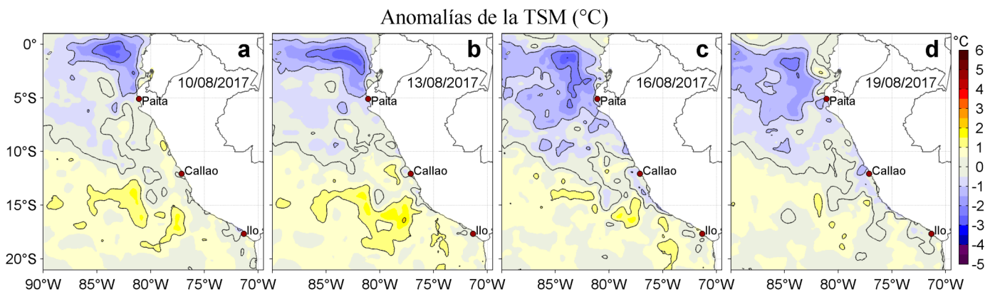
Figura 3. Anomalías de la Temperatura Superficial del Mar ( ^{\circ}\text{C} ) para los días: a) 10, b) 13, c) 16, y d) 19 de agosto de 2017. Las anomalías se calcularon respecto de la climatología para el periodo 2007-2016. Datos: OSTIA-UKMO-L4-GLOB-v2.0 (UK Met Office, 2012; Donlon et al, 2012). Procesamiento: LHF/AFIOF/DGIOCC/IMARPE.
