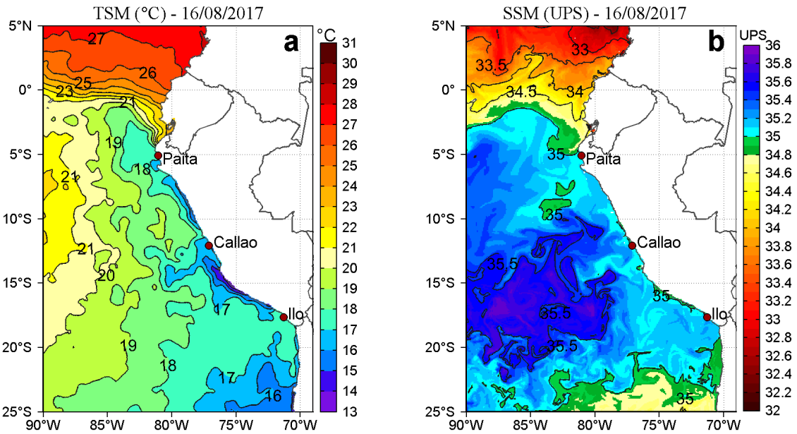
Figura 2. a) Temperatura superficial del mar (°C) y b) Salinidad superficial del mar (UPS) para el 16 de agosto respectivamente. Datos: OSTIA-UKMO-L4-GLOB-v2.0 (UK Met Office, 2012; Donlon et al, 2012) disponible en https://podaac.jpl.nasa.gov/dataset/OSTIA-UKMO-L4-GLOB-v2.0 para (a) y Hybrid Coordinate Ocean Model (HYCOM; Halliwell et al., 1998; 2000; Bleck, 2001) para (b). Procesamiento: LHF/AFIOF/DGIOCC/IMARPE.
