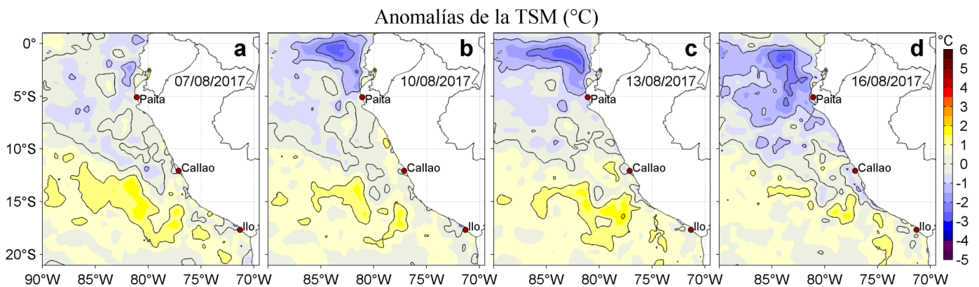
Figura 3. Anomalías de la Temperatura Superficial del Mar (°C) para los días: a) 07, b) 10, c) 13, y d) 16 de agosto de 2017. Las anomalías se calcularon respecto de la climatología para el periodo 2007-2016. Datos: OSTIA-UKMO-L4-GLOB-v2.0 (UK Met Office, 2012; Donlon et al, 2012). Procesamiento: LHF/AFIOF/DGIOCC/IMARPE.
