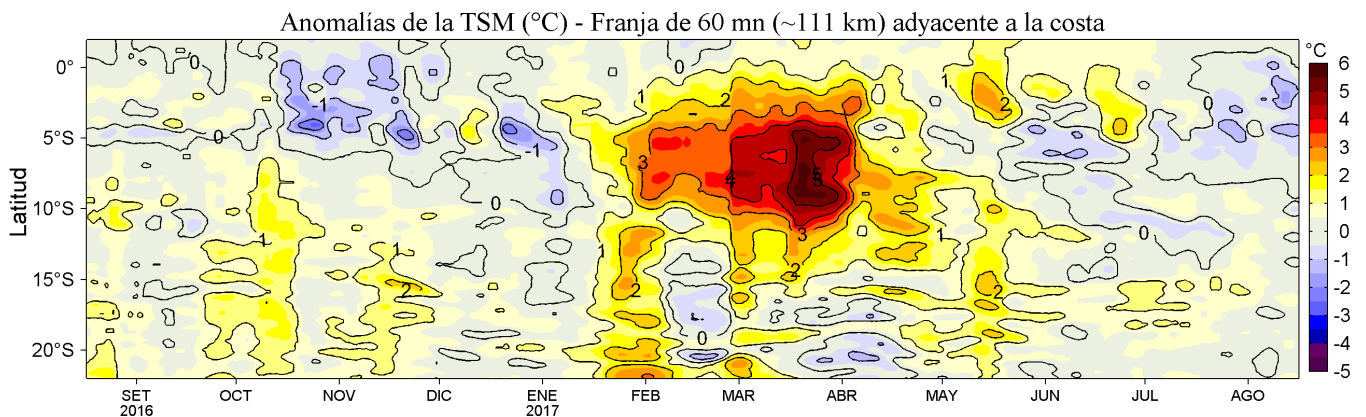
Figura 4. Variación promedio de las anomalías de la temperatura superficial del mar (°C) para una franja de 60 mn (~111 km) adyacente al litoral peruano para los últimos doce meses al 16 de agosto de 2017. Se distingue el calentamiento ocurrido de mediados de enero a fines de mayo de 2017 asociado con la presencia de El Niño Costero, evento que tuvo mayor impacto en la TSM (+5°C) en la segunda quincena de marzo. Datos: OSTIA-UKMO-L4-GLOB-v2.0 (UK Met Office, 2012; Donlon et al, 2012) disponible en https://podaac.jpl.nasa.gov/dataset/OSTIA-UKMO-L4-GLOB-v2.0 . Las anomalías se calcularon con respecto al periodo 2007-2016. Procesamiento: LHF/AFIOF/DGIOCC/IMARPE.
