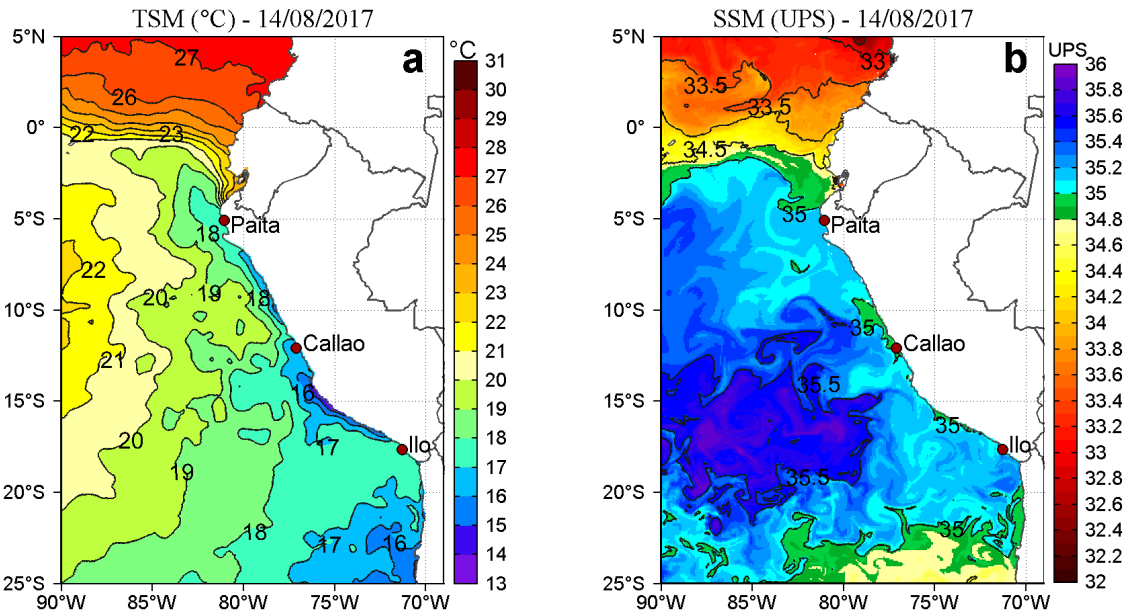
Figura 2. a) Temperatura superficial del mar ( ^{\circ}\text{C} ) y b) Salinidad superficial del mar (UPS) para el 14 de agosto respectivamente. Datos: OSTIA-UKMO-L4-GLOB-v2.0 (UK Met Office, 2012; Donlon et al, 2012) disponible en https://podaac.jpl.nasa.gov/dataset/OSTIA-UKMO-L4-GLOB-v2.0 para (a) y Hybrid Coordinate Ocean Model (HYCOM; Halliwell et al., 1998; 2000; Bleck, 2001) para (b). Procesamiento: LHF/AFIOF/DGIOCC/IMARPE.
