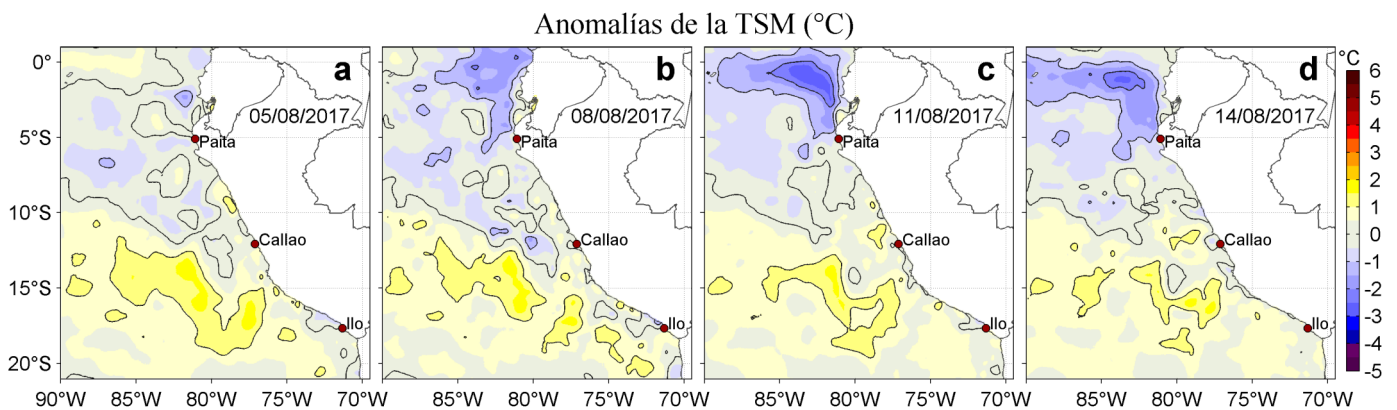
Figura 3. Anomalías de la Temperatura Superficial del Mar ( ^{\circ}\text{C} ) para los días: a) 05, b) 08, c) 11, y d) 14 de agosto de 2017. Las anomalías se calcularon respecto de la climatología para el periodo 2007-2016. Datos: OSTIA-UKMO-L4-GLOB-v2.0 (UK Met Office, 2012; Donlon et al, 2012). Procesamiento: LHF/AFIOF/DGIOCC/IMARPE.
